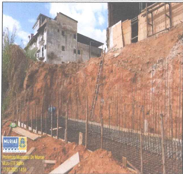
Montagem de Ferragem Estrutura do Muro
