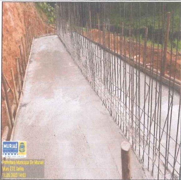
concreto Usinado Bombeado 25 Mpa Estrutura do Muro
