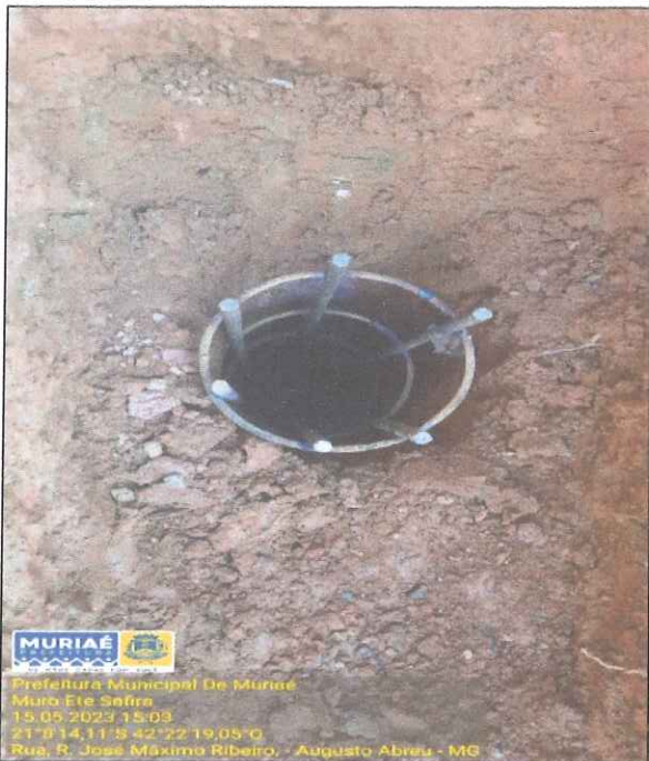
Armadura estaca D= 20cm CA- 6.3mm 10.00mm
