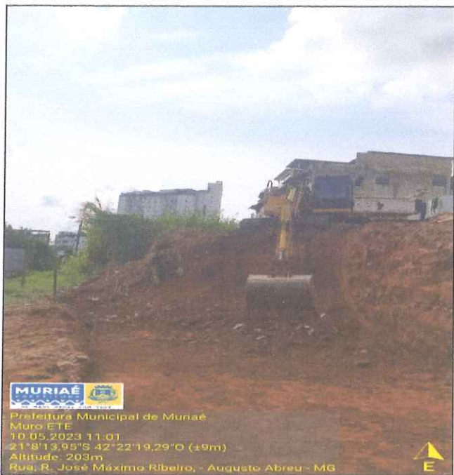
Escavação mecanizada
