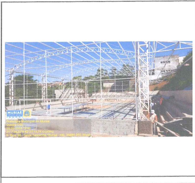
Foto 1: EXECUÇÃO DA ALVENARIA, CHAPISCO E REVESTIMENTO EM ARGAMASSA DA MURETA.
