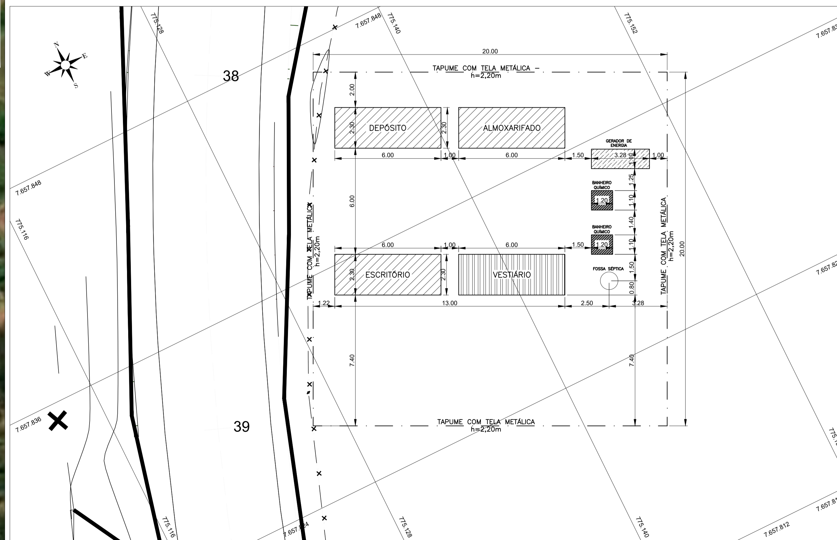
CANTEIRO DE OBRAS ESCALA 1:125
