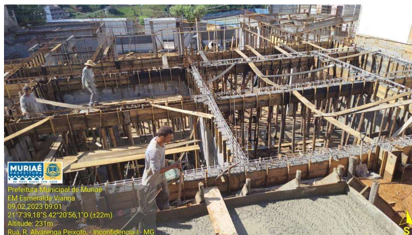
Imagem 14: concretagem das vigas Fonte: arquivo próprio equipe fiscalização
