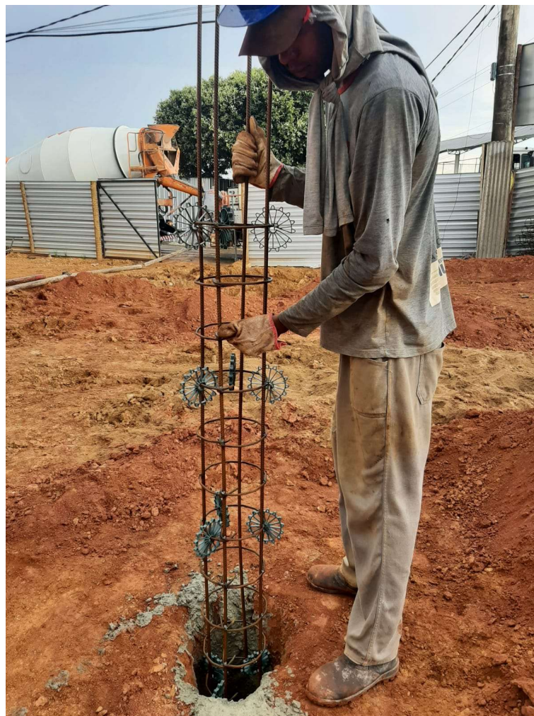
Imagem 06: armação de estaca Fonte: arquivo próprio equipe fiscalização
