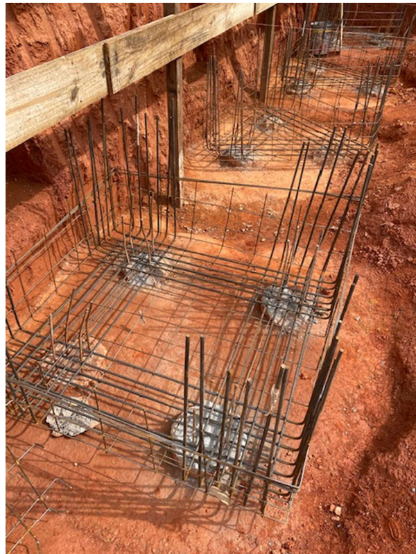
Imagem 09: armação dos blocos de coroamento
