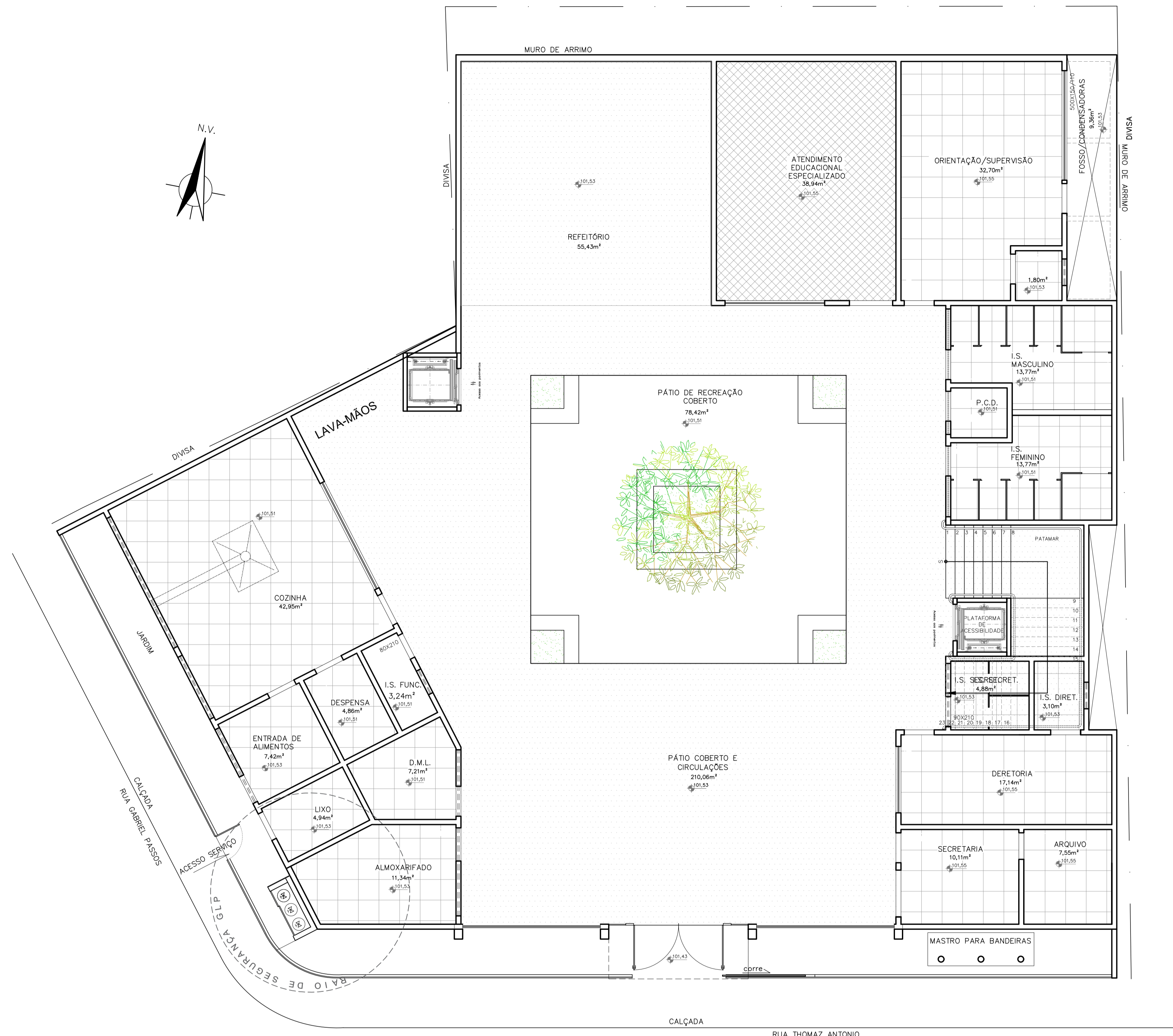
PLANTA TETO 1º PAVIMENTO ESCALA 1:75 ACESSO RUA THOMAZ ANTONIO
