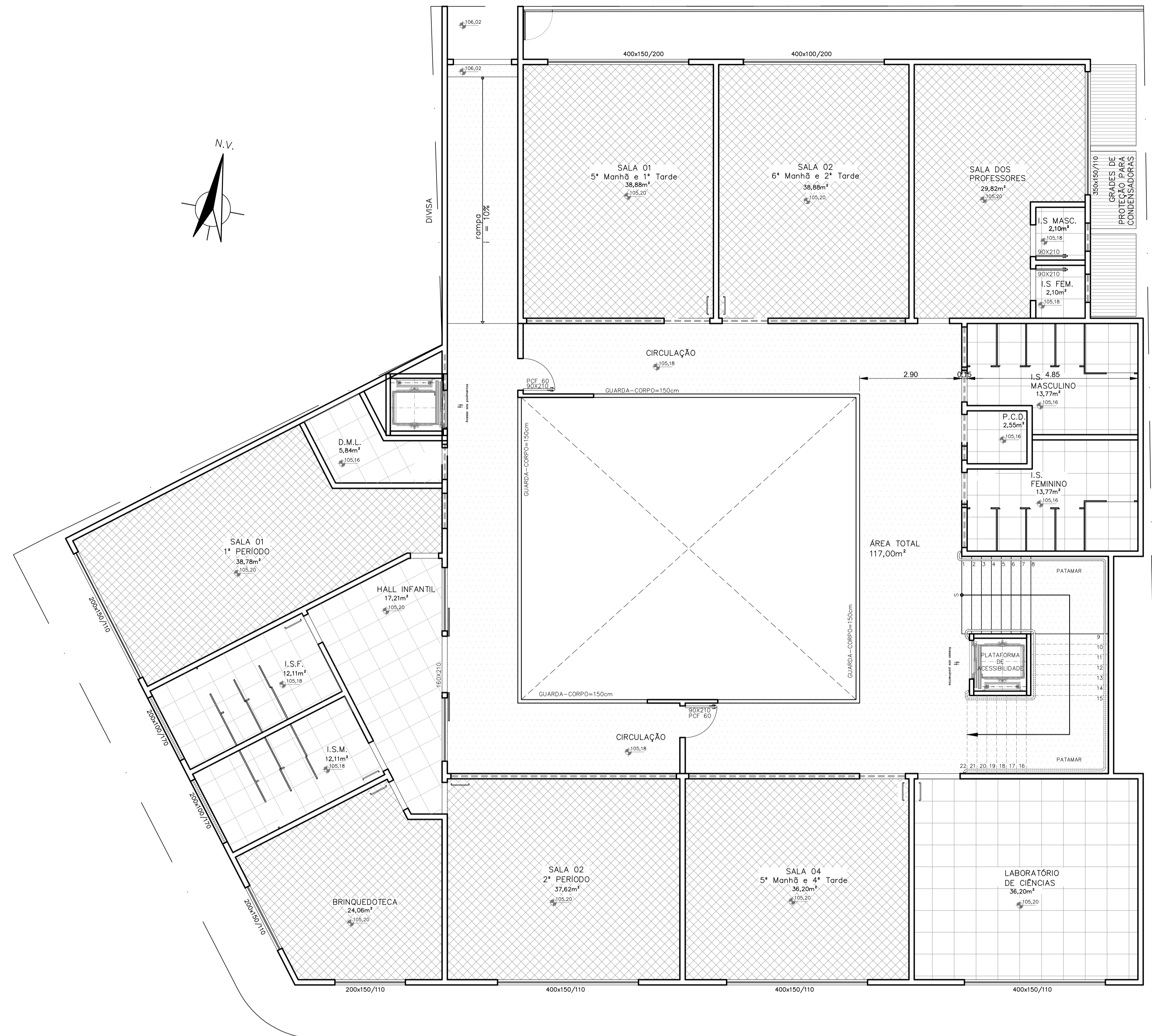
PLANTA TETO 2º PAVIMENTO ESCALA 1:75 ACESSO RUA ALVARENGA PEIXOTO
