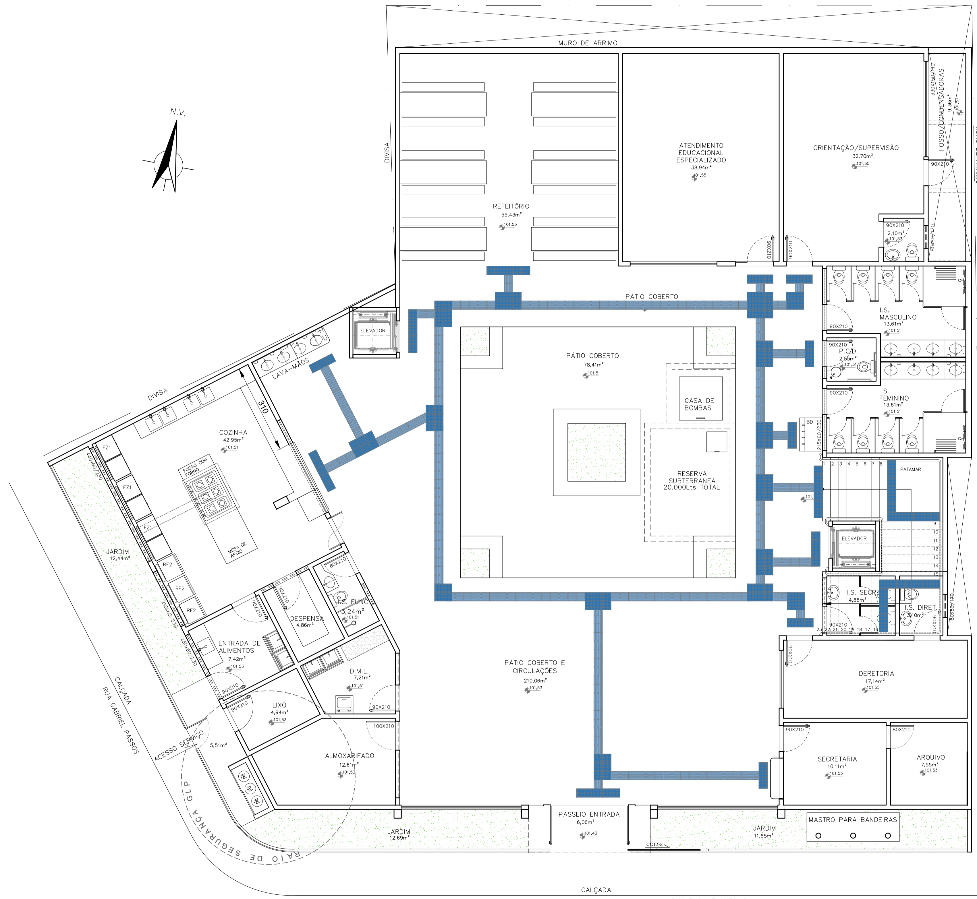
PLANTA ACESSIBILIDADE 1º PAVIMENTO ESCALA 1:75 ACESSO RUA THOMAZ ANTONIO
