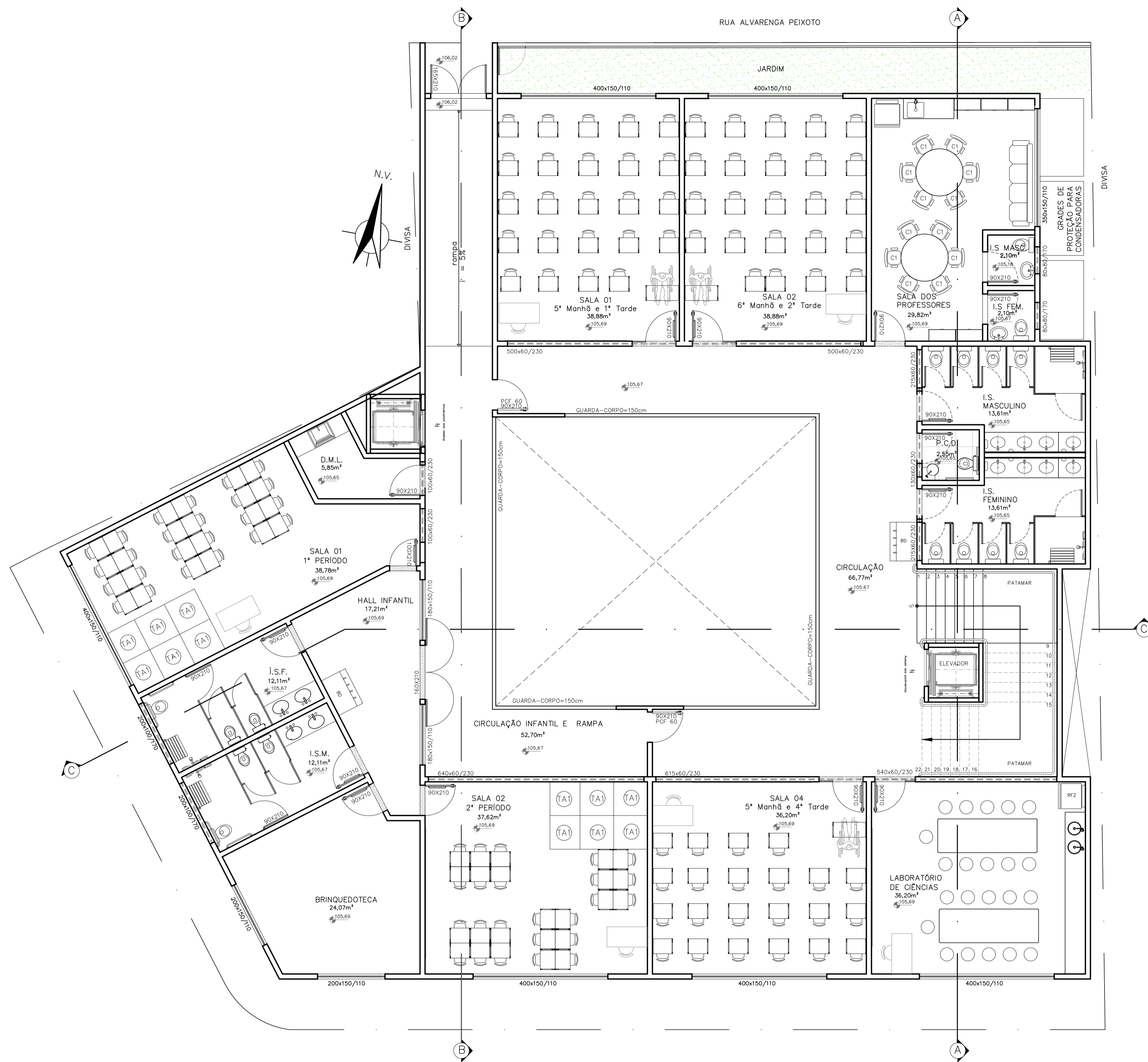
PLANTA LAYOUT 2º PAVIMENTO ESCALA 1:75 ACESSO RUA ALVARENGA PEIXOTO
