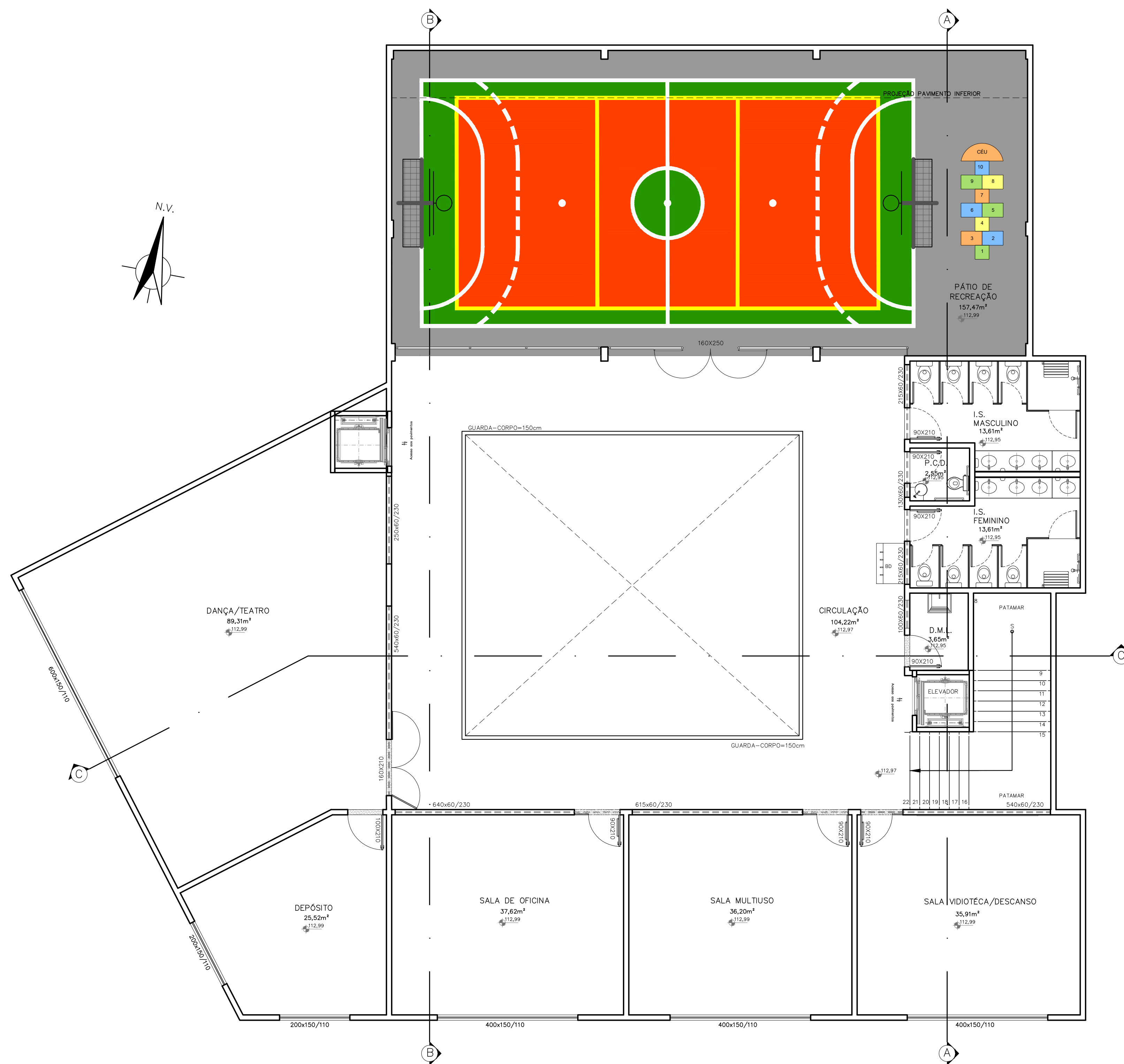
PLANTA LAYOUT 4º PAVIMENTO ESCALA 1:75
