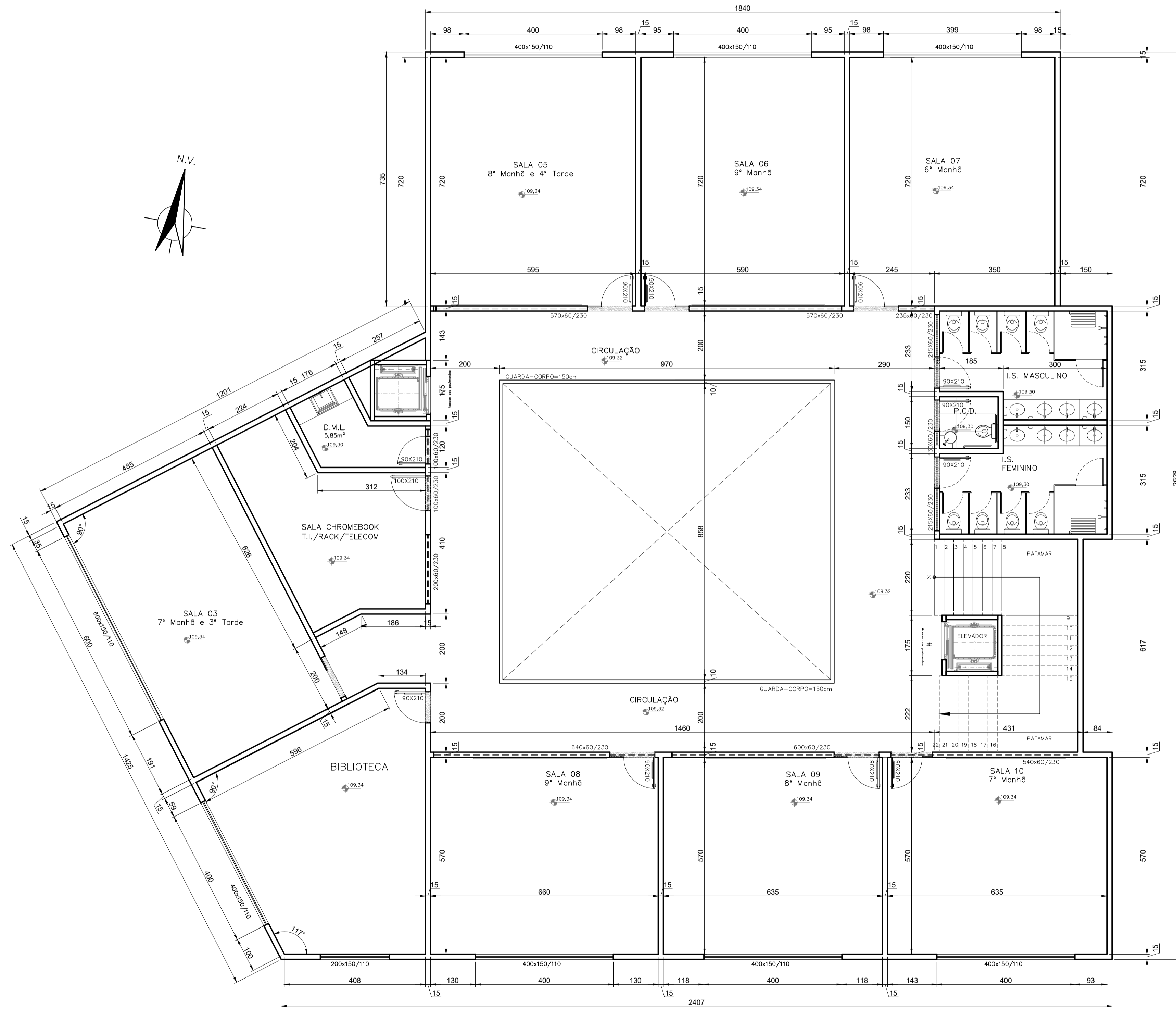
PLANTA DE DIMENSIONAMENTO 3º PAVIMENTO ESCALA 1:75
