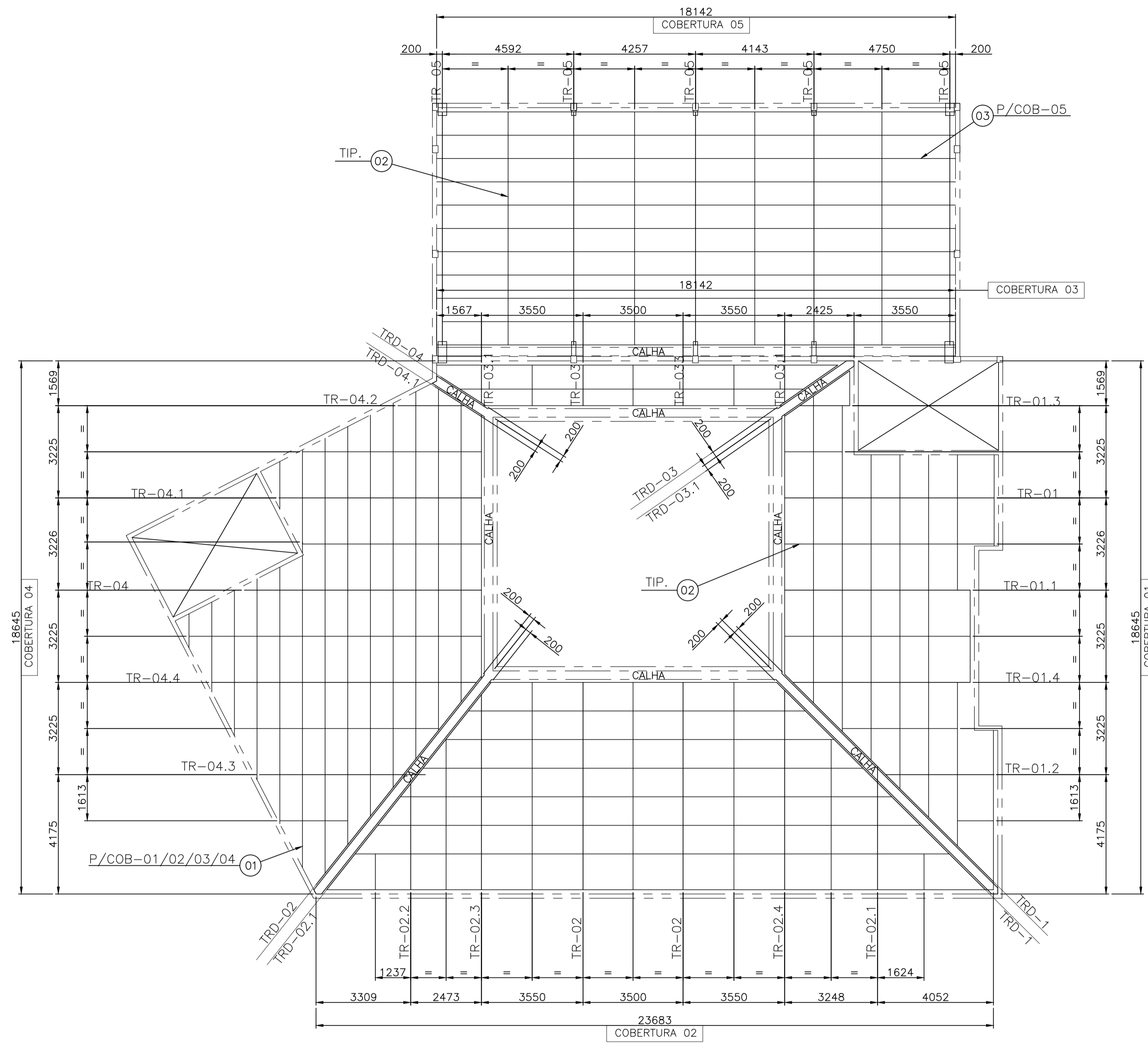
PLANO DAS TERÇAS E TRELIÇAS CESALA: 1/125
