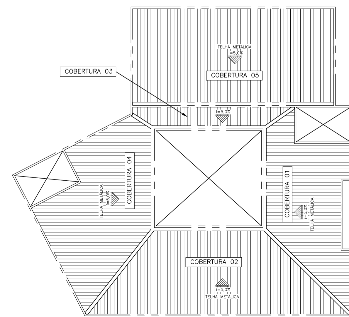
PLANTA CHAVE DAS COBERTURAS
