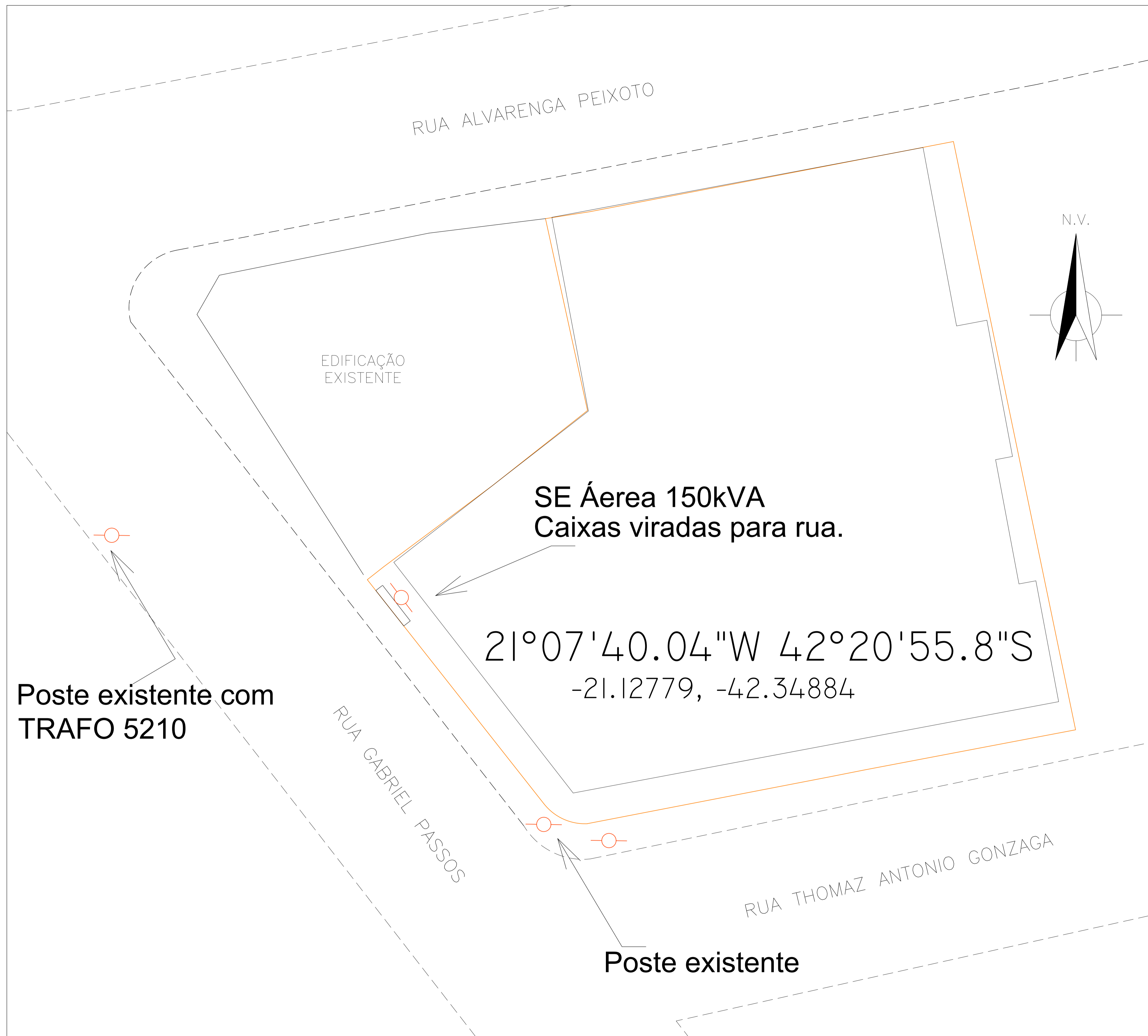
PLANTA DE SITUAÇÃO - ESCOLA MUNICIPAL PROFESSORA ESMERALDA VIANA ESCALA 1:100
