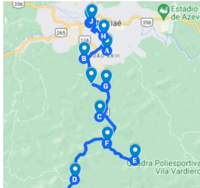
Imagem 1: Projeto Básico da linha Muriaé - Gameleira - Barra Alegre
