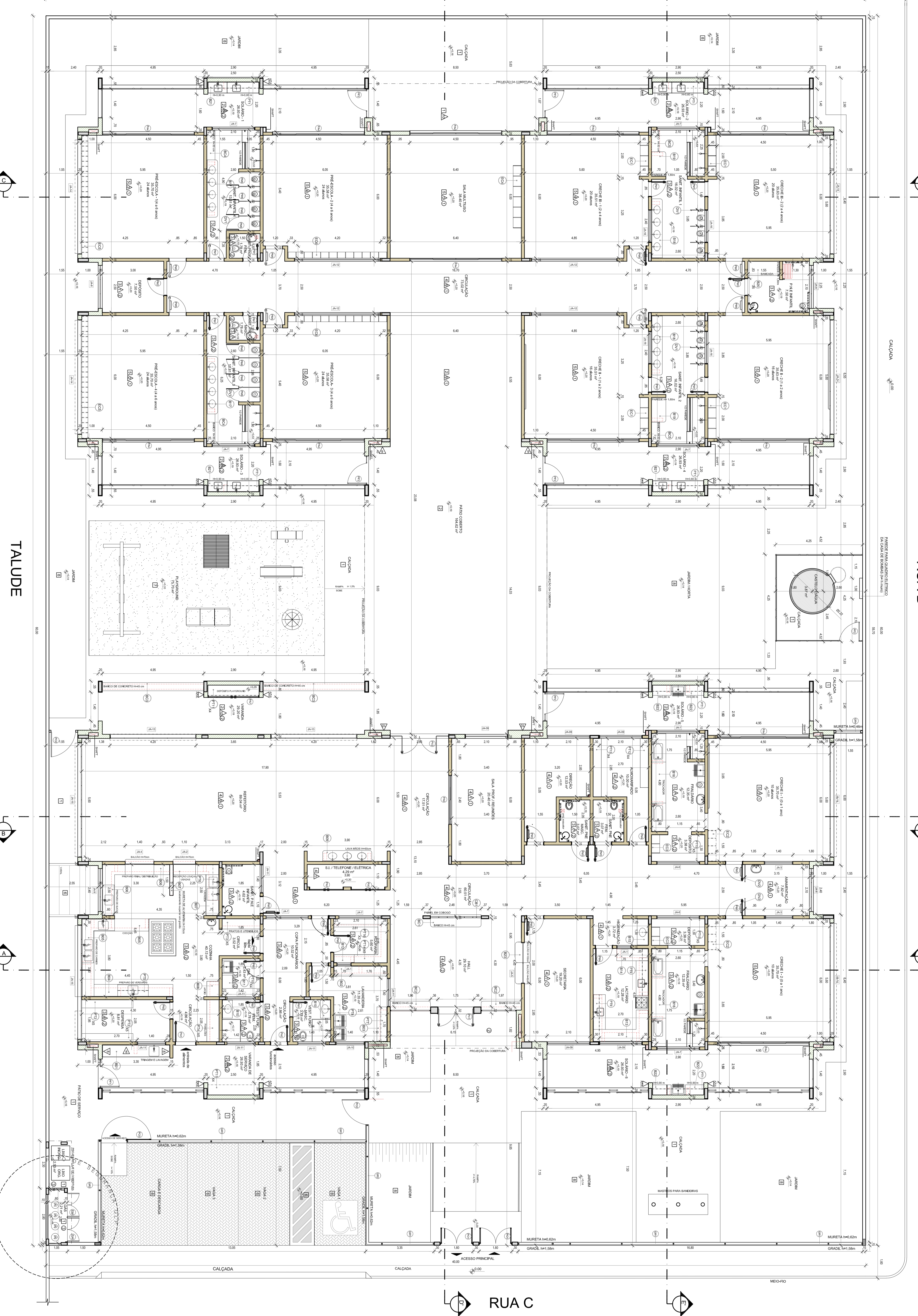
01 PLANTA BAIXA ESC.: 1/75
