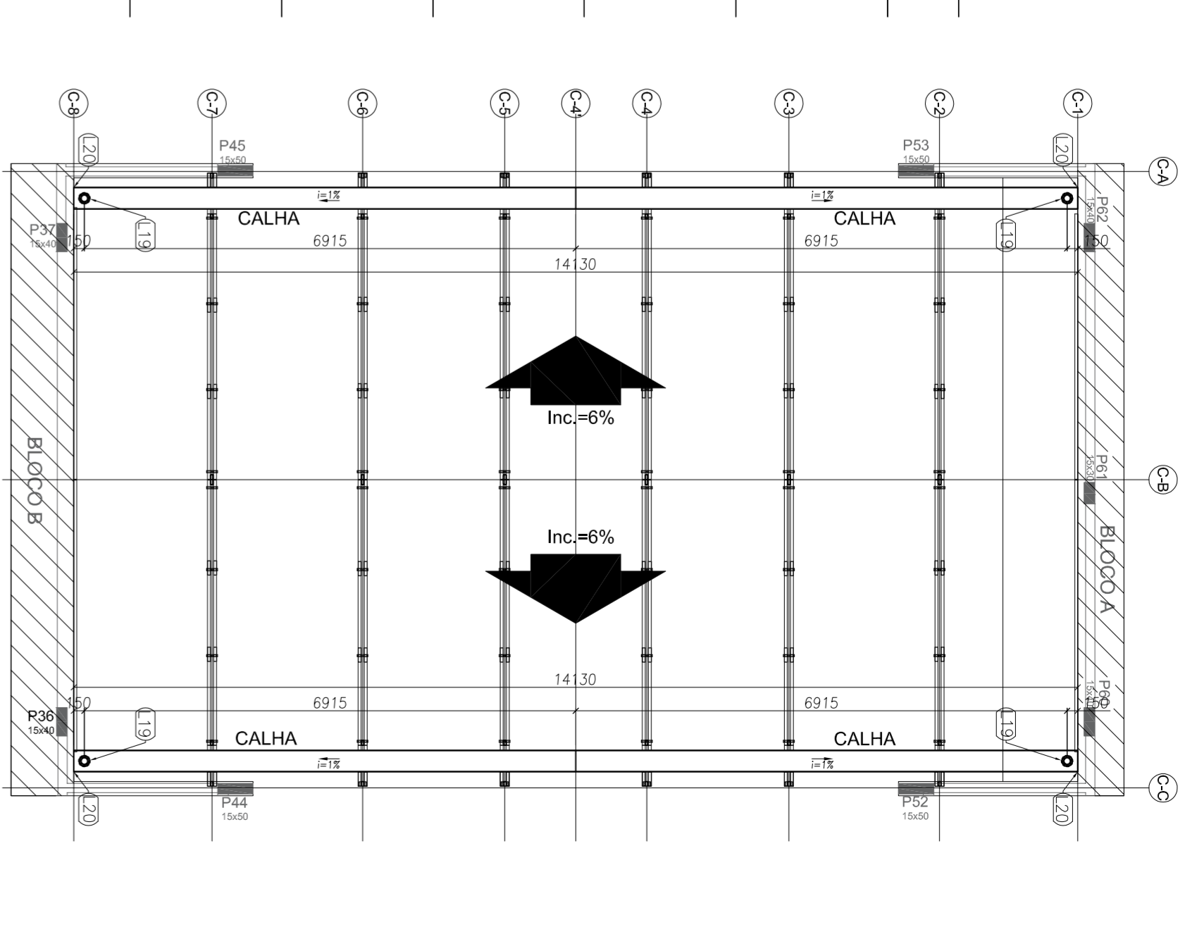
3 BLOCO C - CALHAS ESCALA: 1/75
