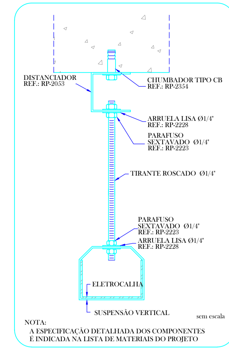
DETALHE TÍPICO DA SUPORTAÇÃO ELETROCALHA - SUSPENSÃO VERTICAL FIXAÇÃO SIMPLES
