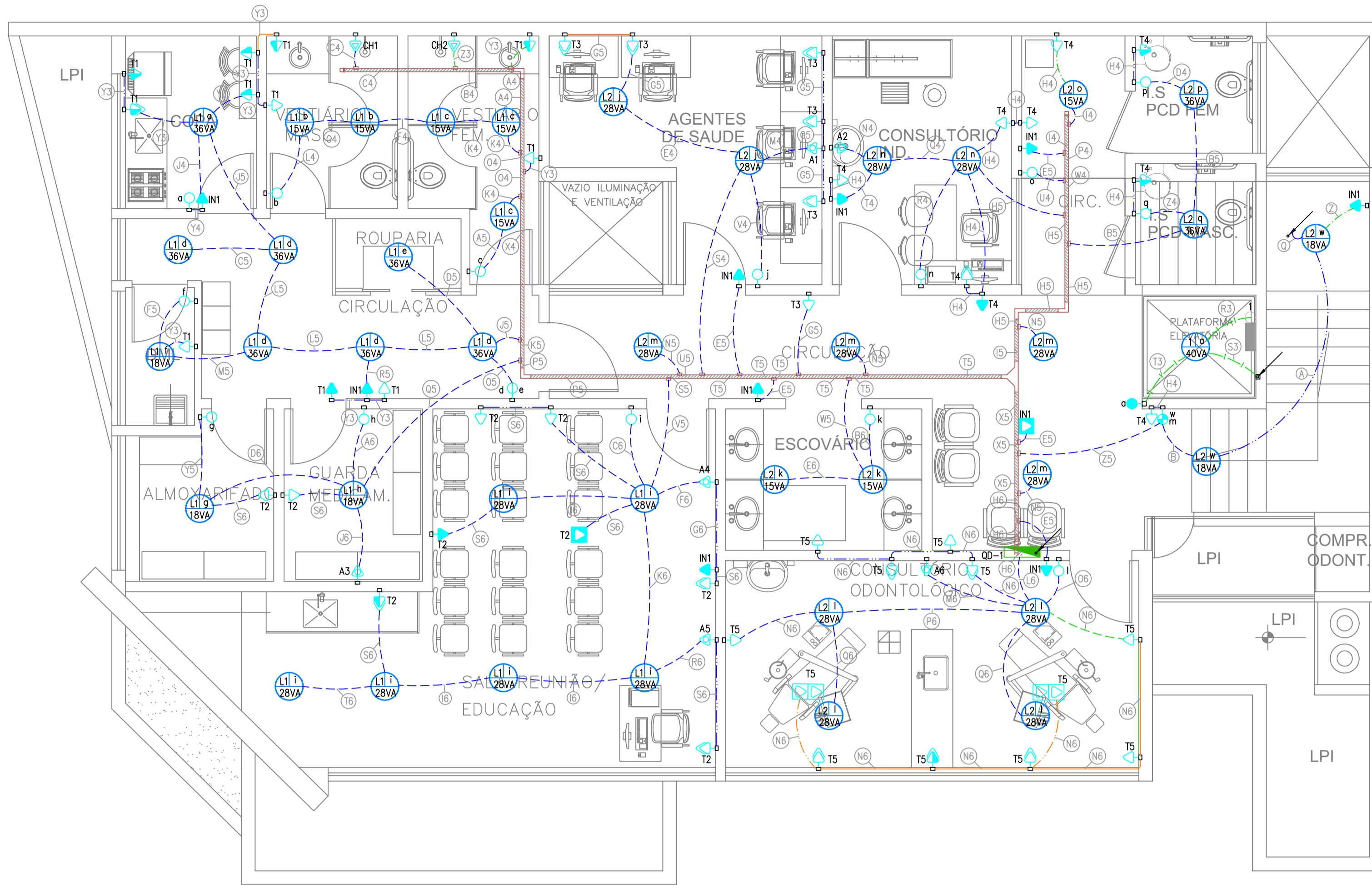
PLANTA BAIXA – 1º PAVIMENTO ESCALA: 1/50
