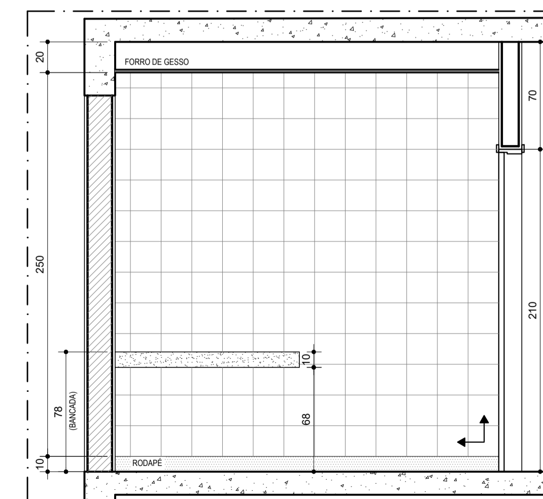
VISTA 04 DETALHE COPA ESCALA.....1/25
