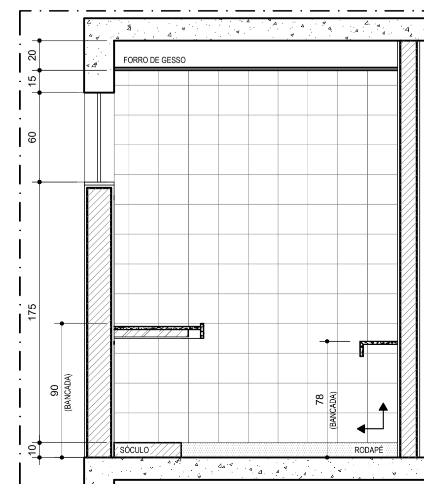
VISTA 03 DETALHE COPA ESCALA.....1/25
