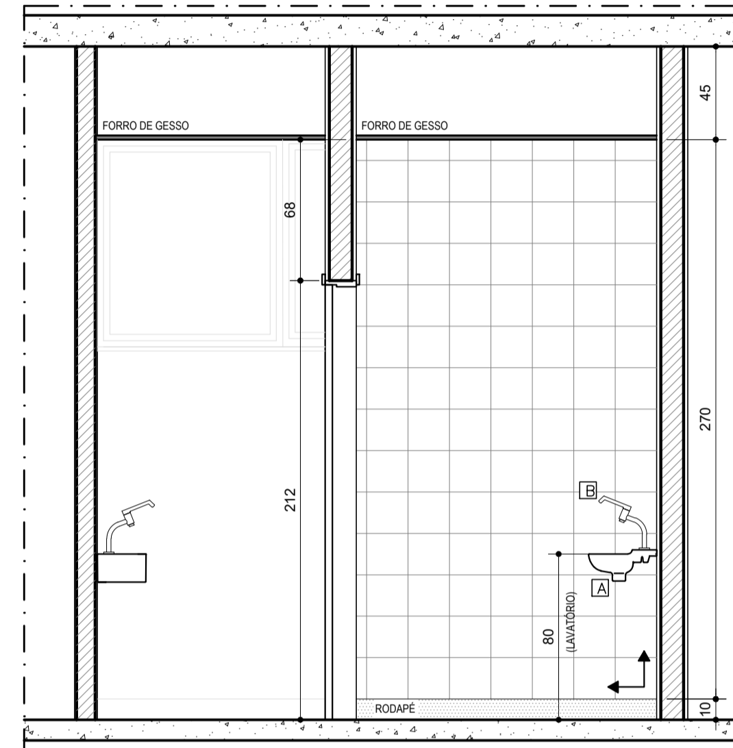
VISTA 01 DETALHE I.S. GINECOLOGIA ESCALA.....1/25
