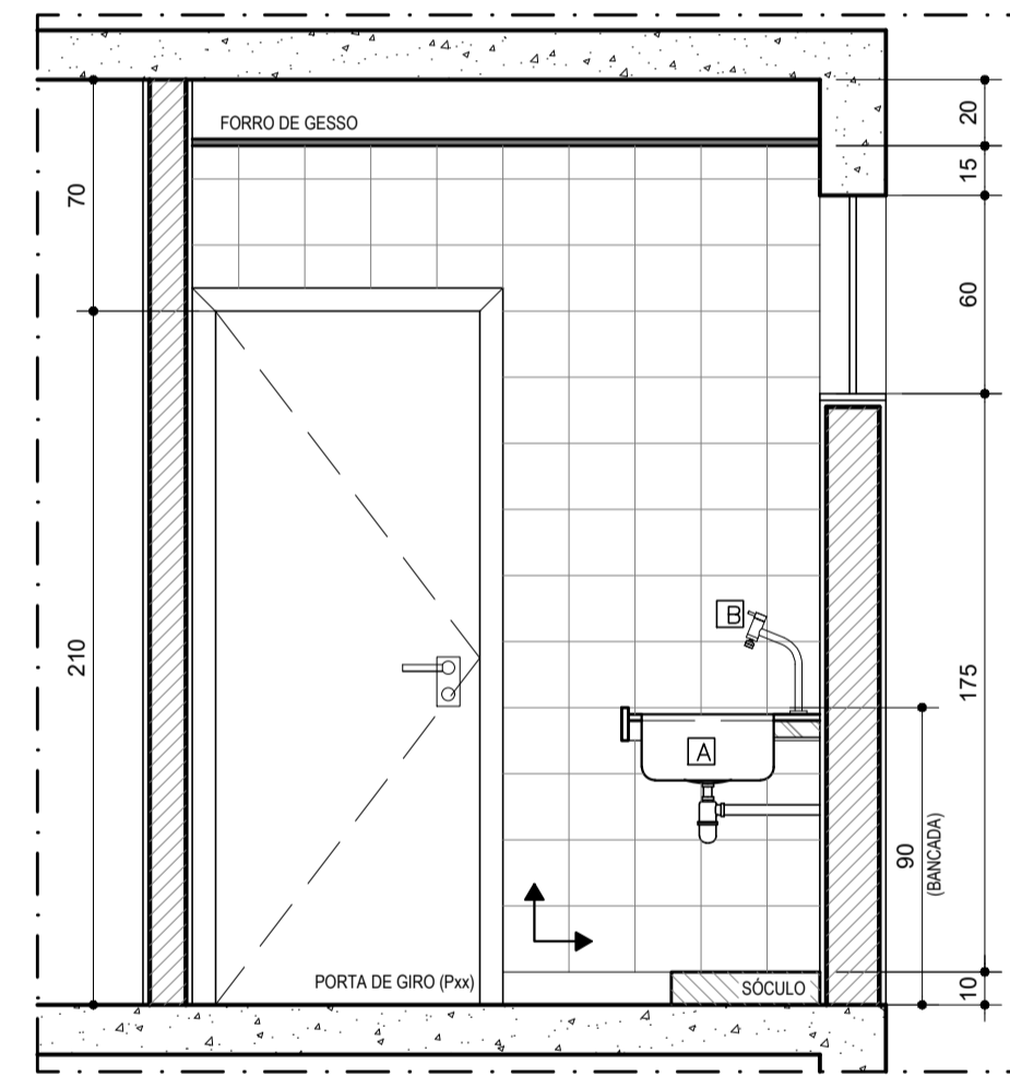
VISTA 01 DETALHE COPA ESCALA.....1/25
