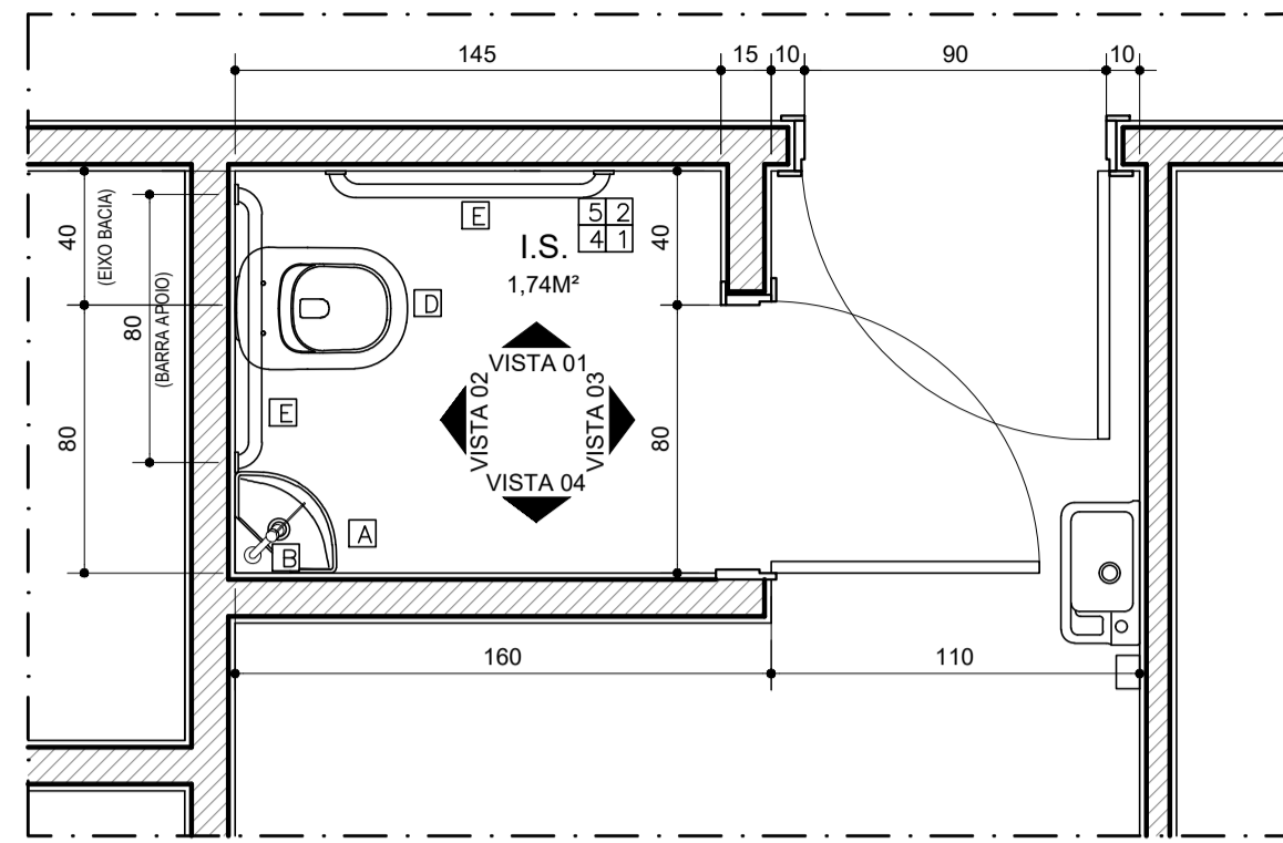
PLANTA DETALHE I.S. GINECOLOGIA ESCALA.....1/25
