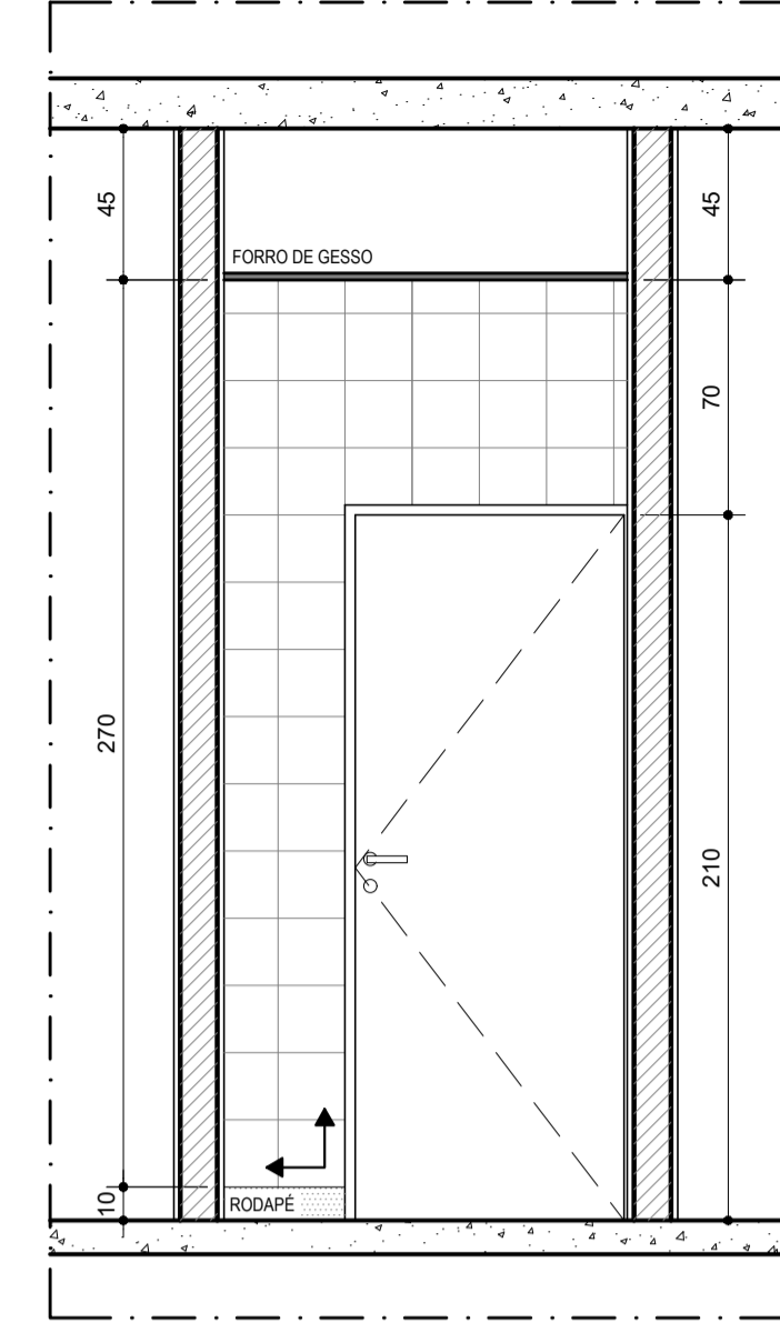
VISTA 03 DETALHE I.S. GINECOLOGIA ESCALA.....1/25
