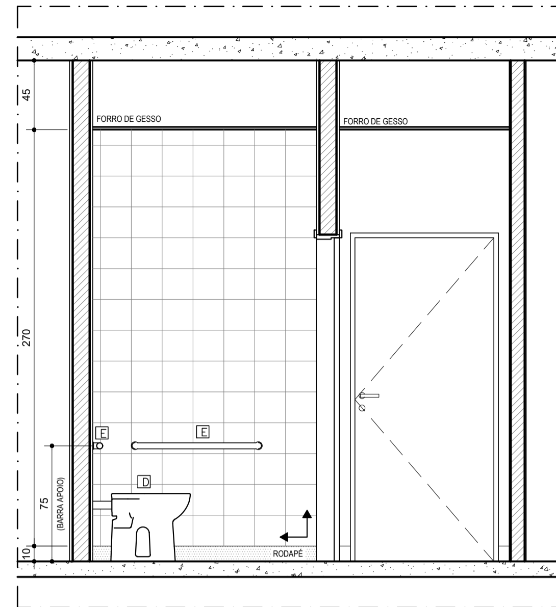
VISTA 02 DETALHE I.S. GINECOLOGIA ESCALA.....1/25
