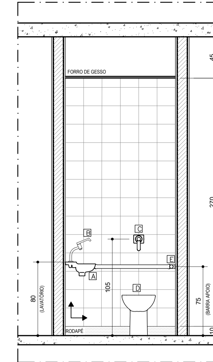
VISTA 04 DETALHE I.S. GINECOLOGIA ESCALA.....1/25
