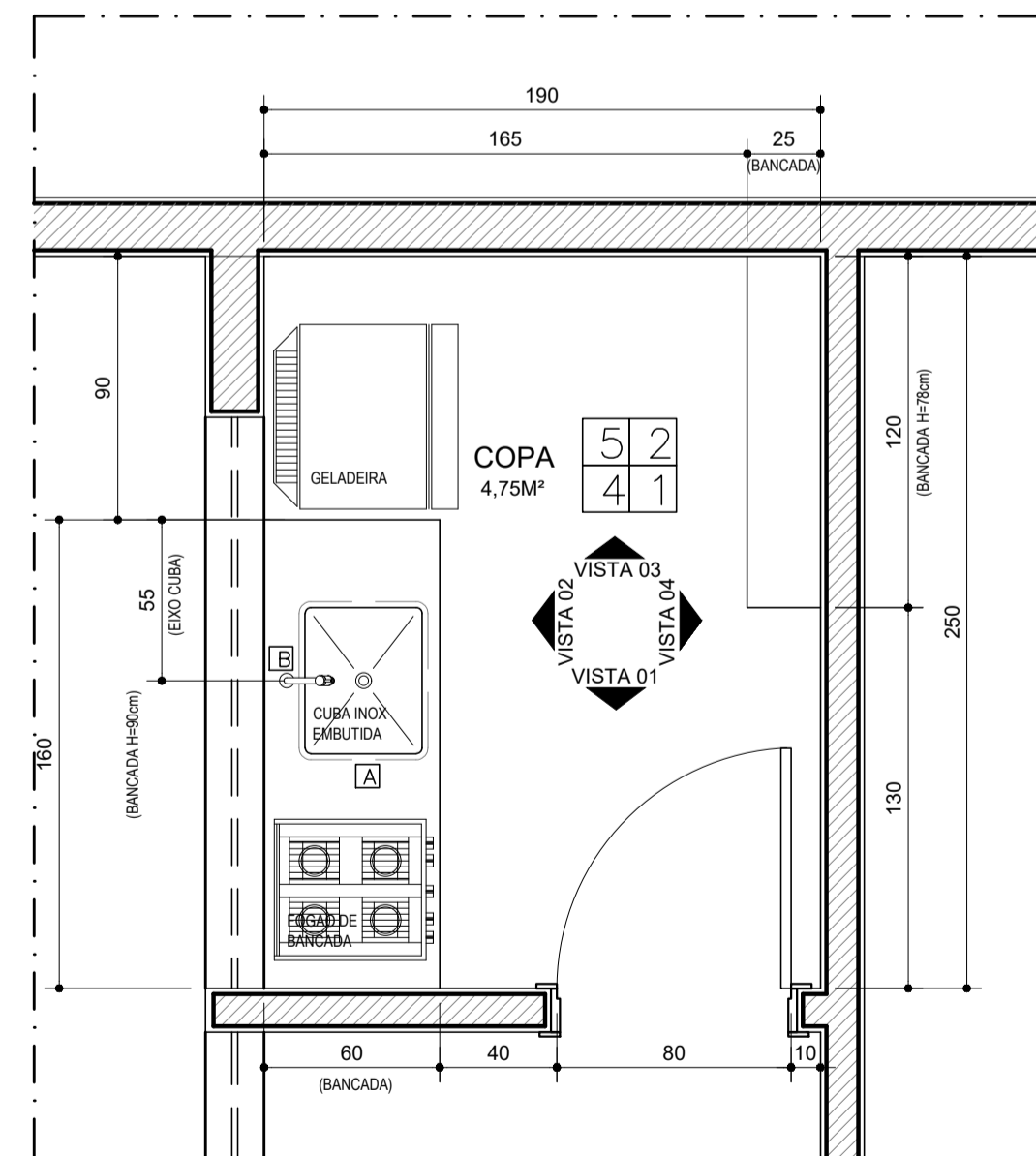
PLANTA DETALHE COPA ESCALA.....1/25
