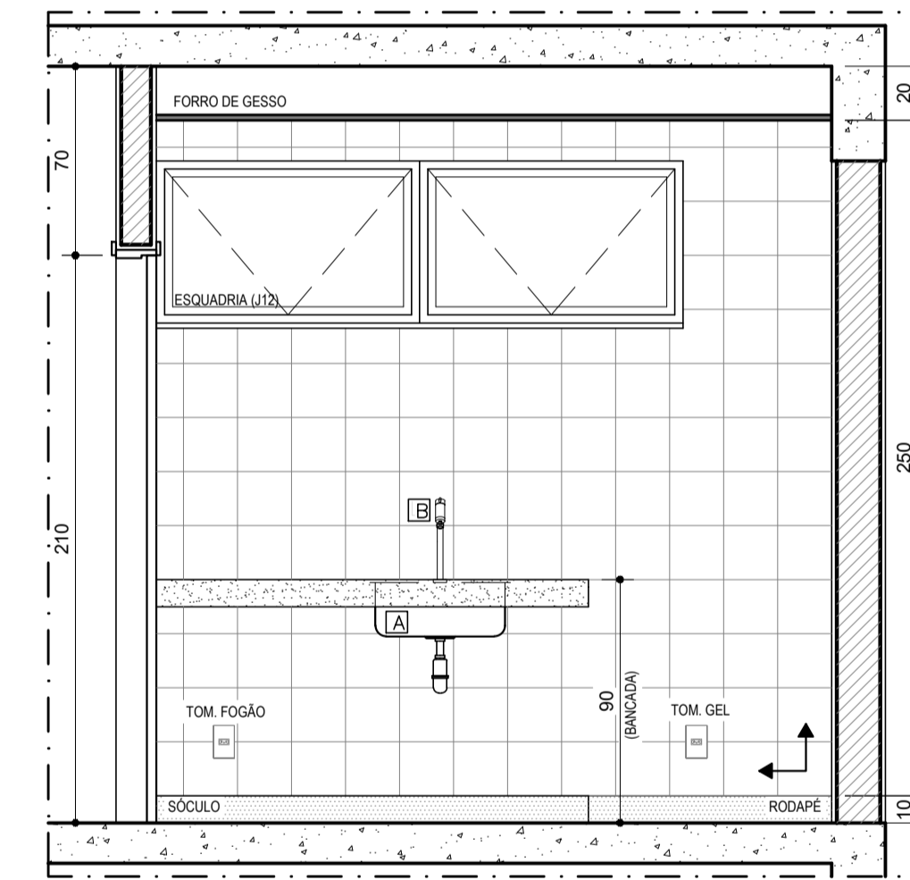
VISTA 02 DETALHE COPA ESCALA.....1/25
