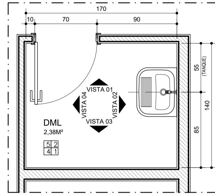
PLANTA DETALHE DML TÉRREO ESCALA.....1/25 OBS: INSTALAR VENTILAÇÃO MECÂNICA TIPO VENTOKIT
