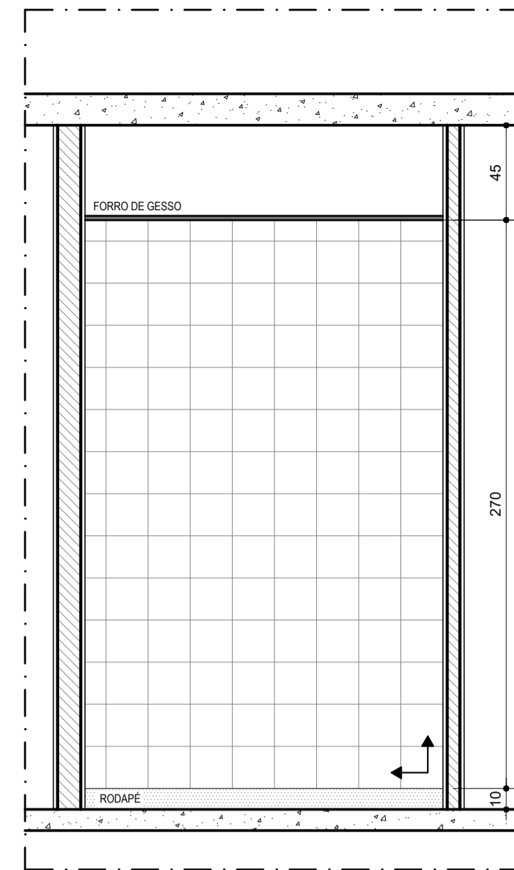
VISTA 03 DETALHE DML TÉRREO ESCALA.....1/25
