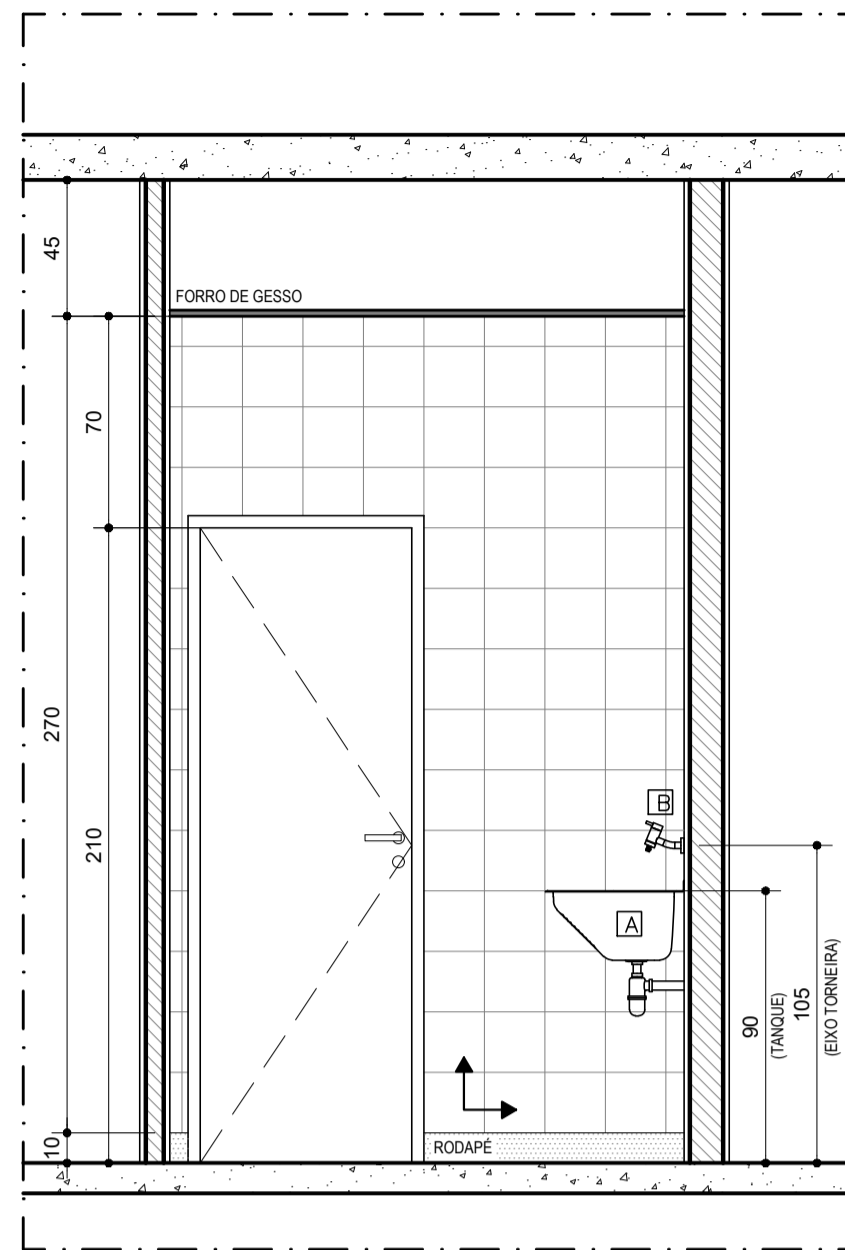
VISTA 01 DETALHE DML TÉRREO ESCALA.....1/25
