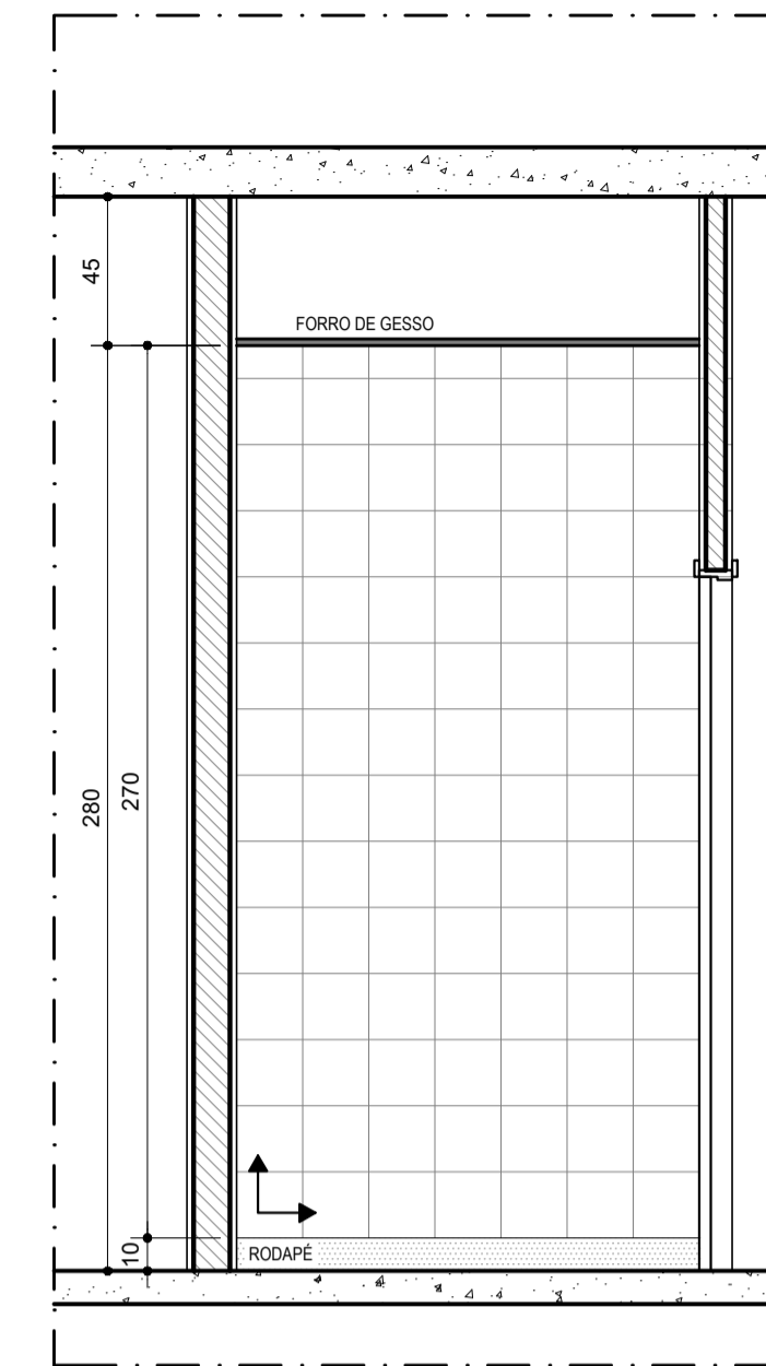
VISTA 03 DETALHE DML TÉRREO ESCALA.....1/25
