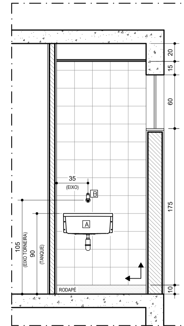
VISTA 03 DETALHE DML 1º PAV. ESCALA.....1/25
