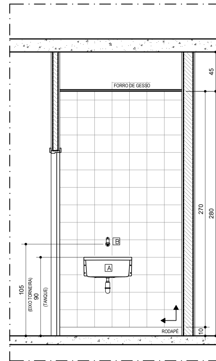
VISTA 02 DETALHE DML TÉRREO ESCALA.....1/25
