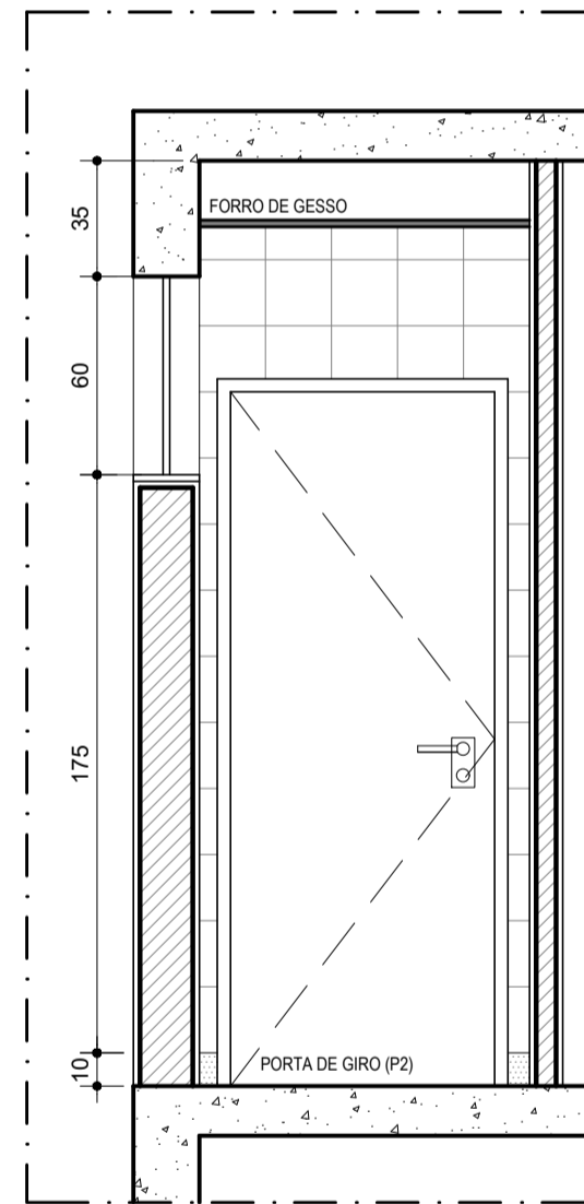
VISTA 01 DETALHE DML 1º PAV. ESCALA.....1/25
