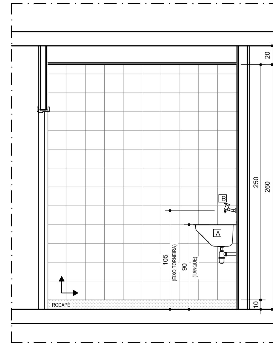
VISTA 02 DETALHE DML 1º PAV. ESCALA.....1/25
