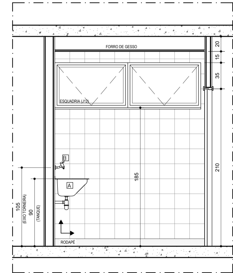
VISTA 04 DETALHE DML 1º PAV. ESCALA.....1/25
