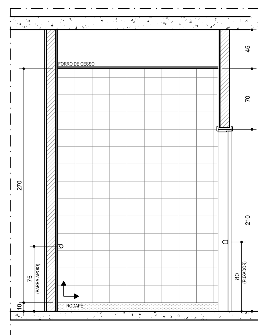
VISTA 04 DETALHE I.S. MASC. TÉRREO ESCALA.....1/25
