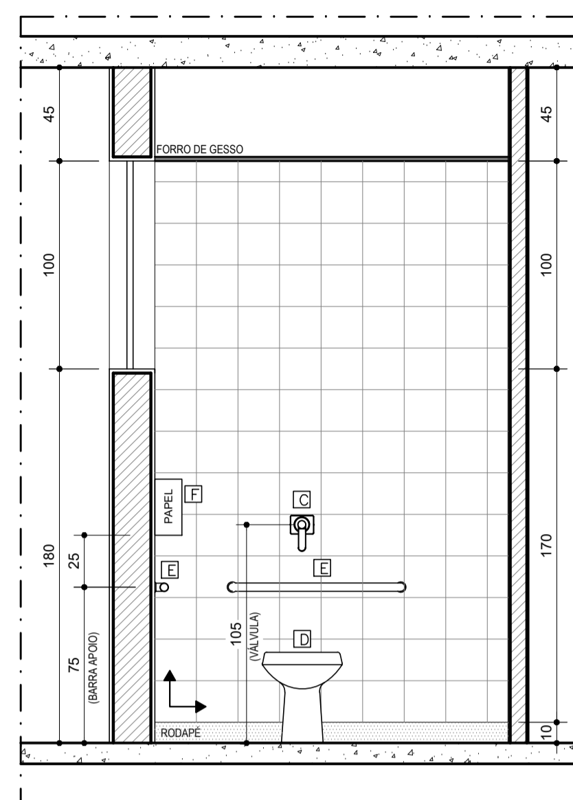
VISTA 01 DETALHE I.S. FEM. TÉRREO ESCALA.....1/25
