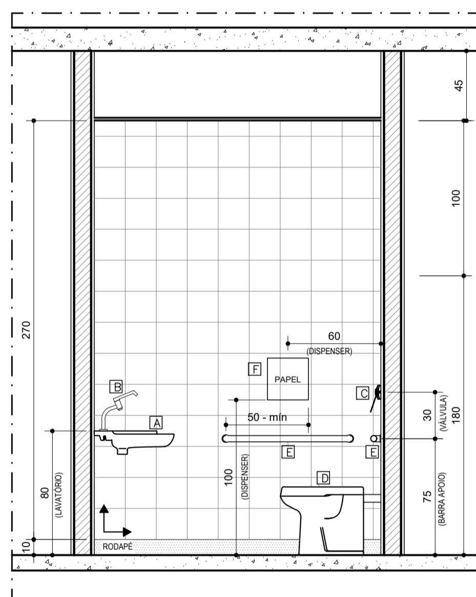
VISTA 02 DETALHE I.S. MASC. TÉRREO ESCALA.....1/25
