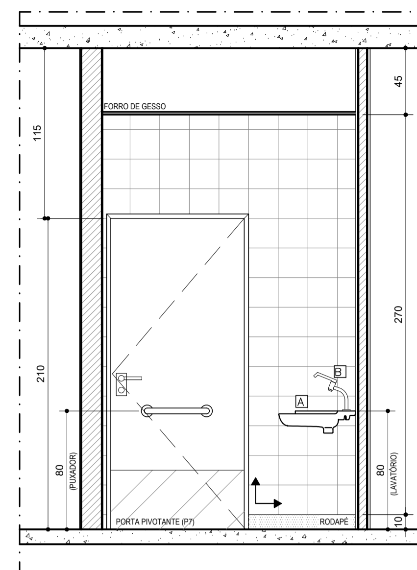
VISTA 01 DETALHE I.S. MASC. TÉRREO ESCALA.....1/25
