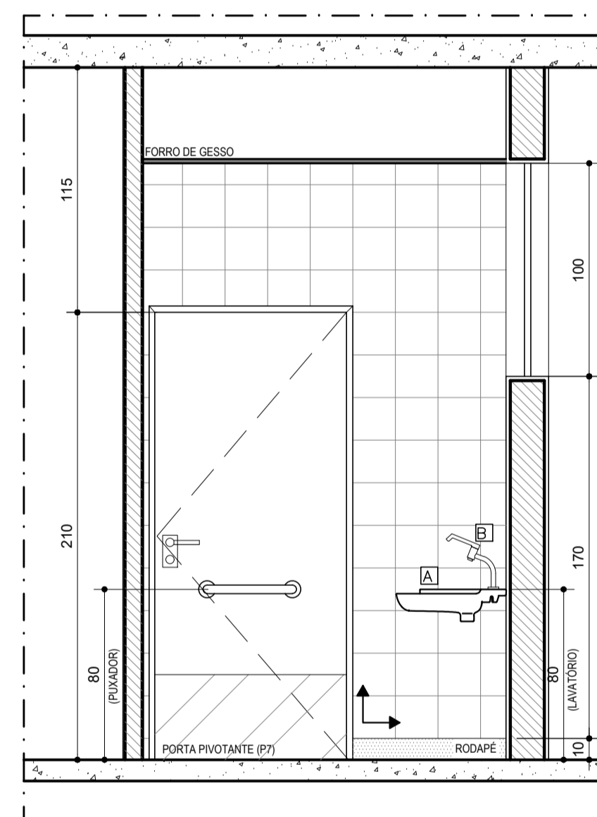
VISTA 03 DETALHE I.S. FEM. TÉRREO ESCALA.....1/25
