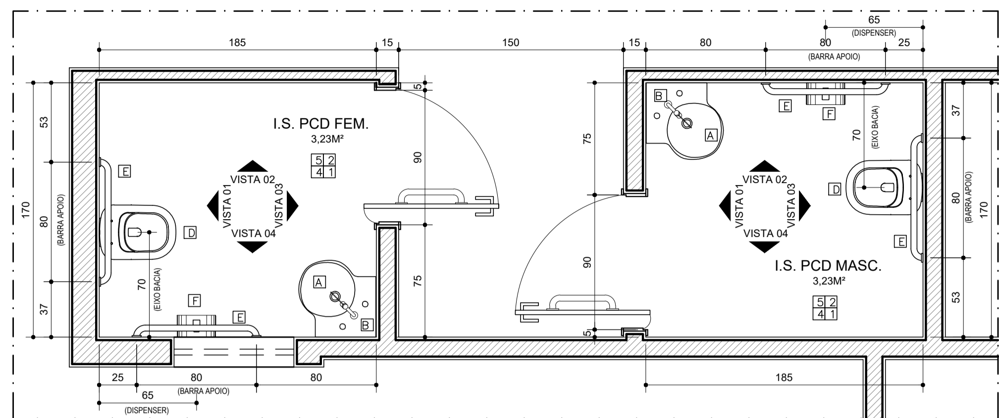
PLANTA DETALHE I.S. FEM / MASC TÉRREO ESCALA.....1/25
