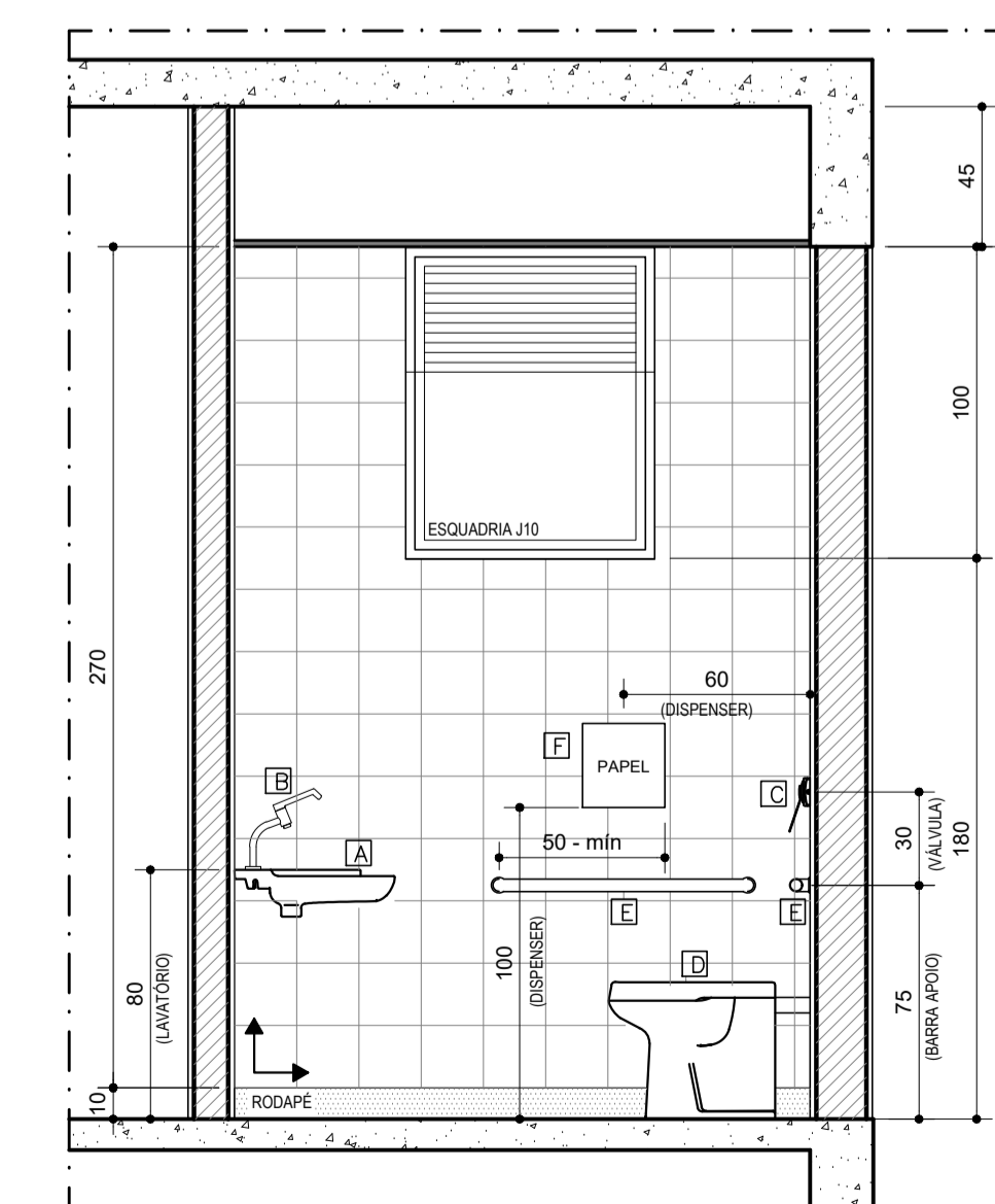
VISTA 04 DETALHE I.S. FEM. TÉRREO ESCALA.....1/25
