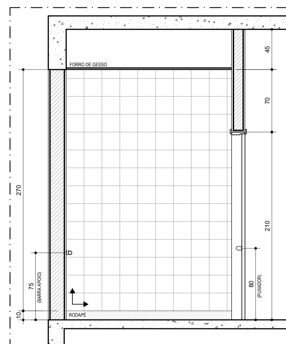
VISTA 02 DETALHE I.S. FEM. TÉRREO ESCALA.....1/25
