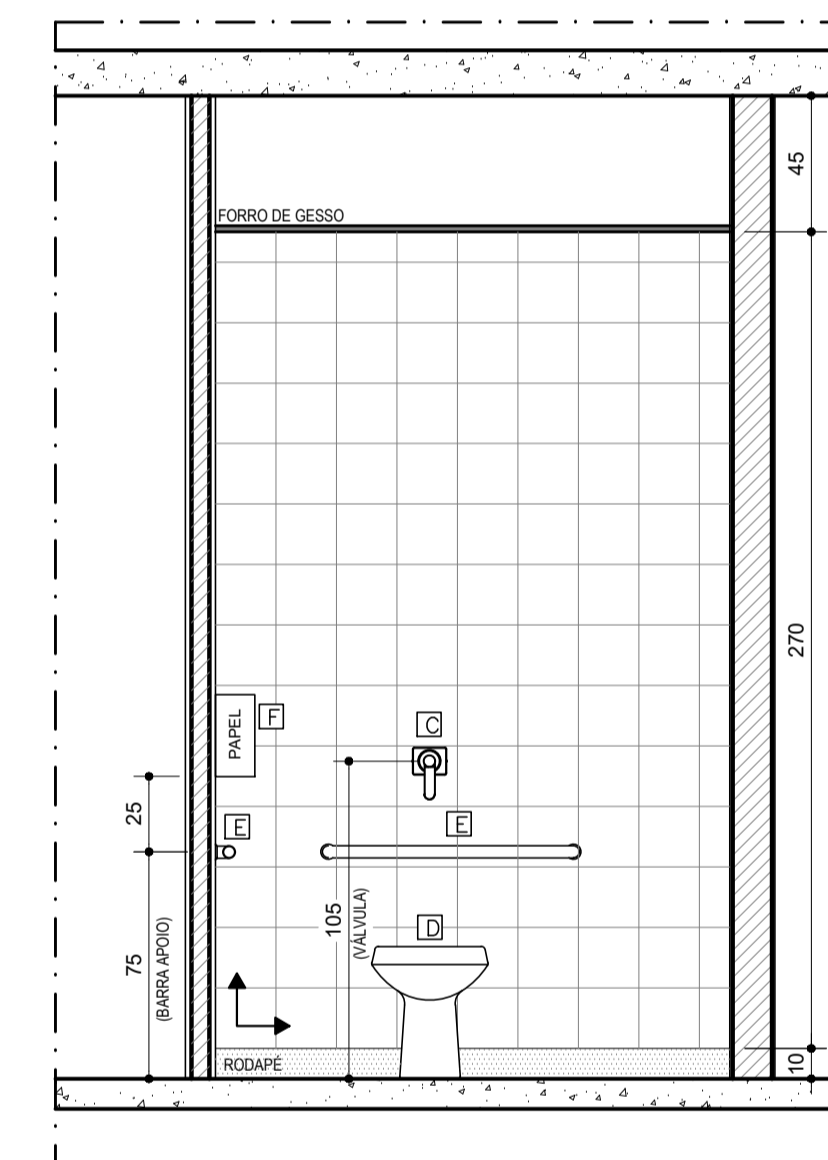
VISTA 03 DETALHE I.S. MASC. TÉRREO ESCALA.....1/25
