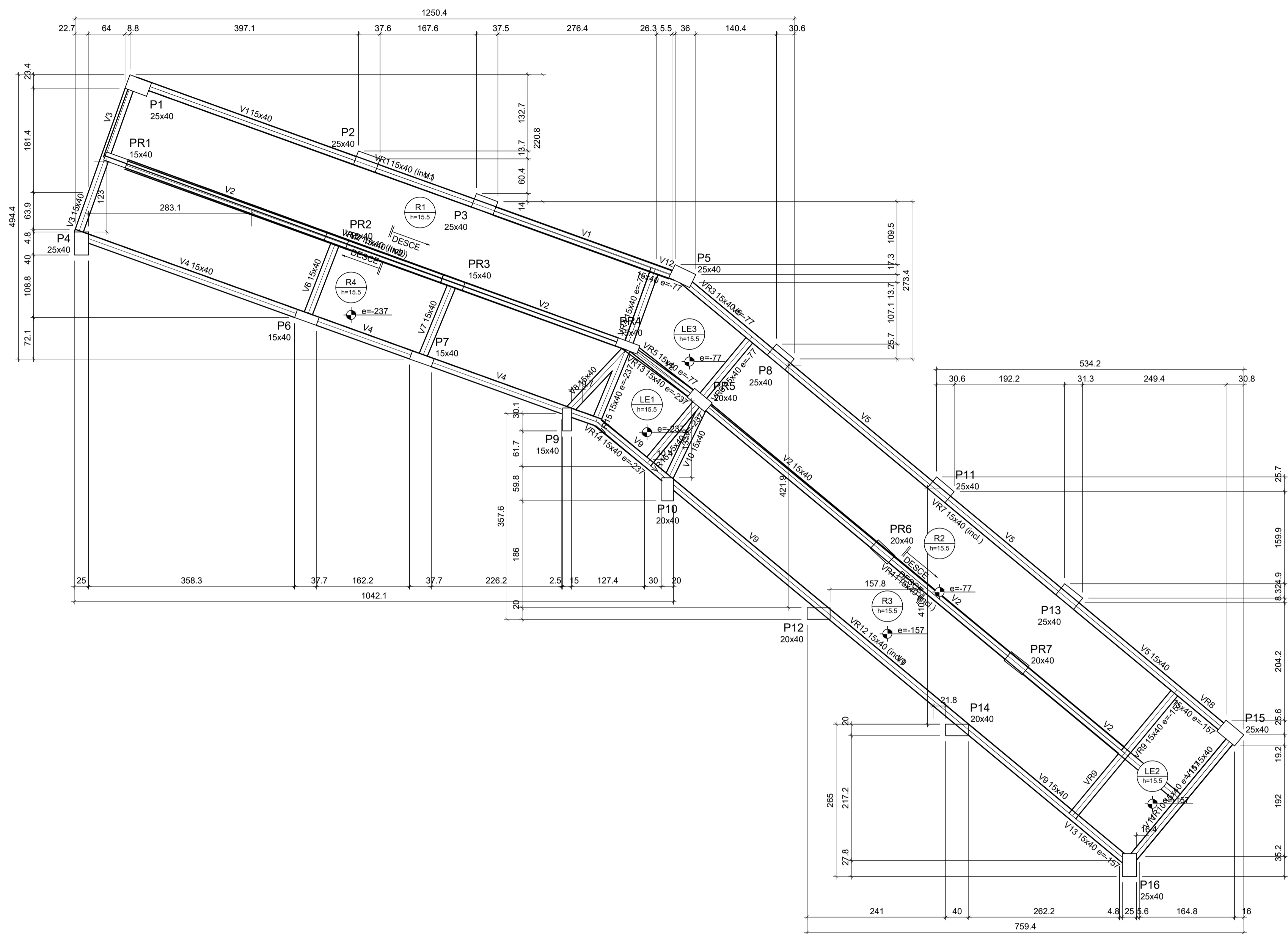
Forma do pavimento Terreo (Nível 342)
