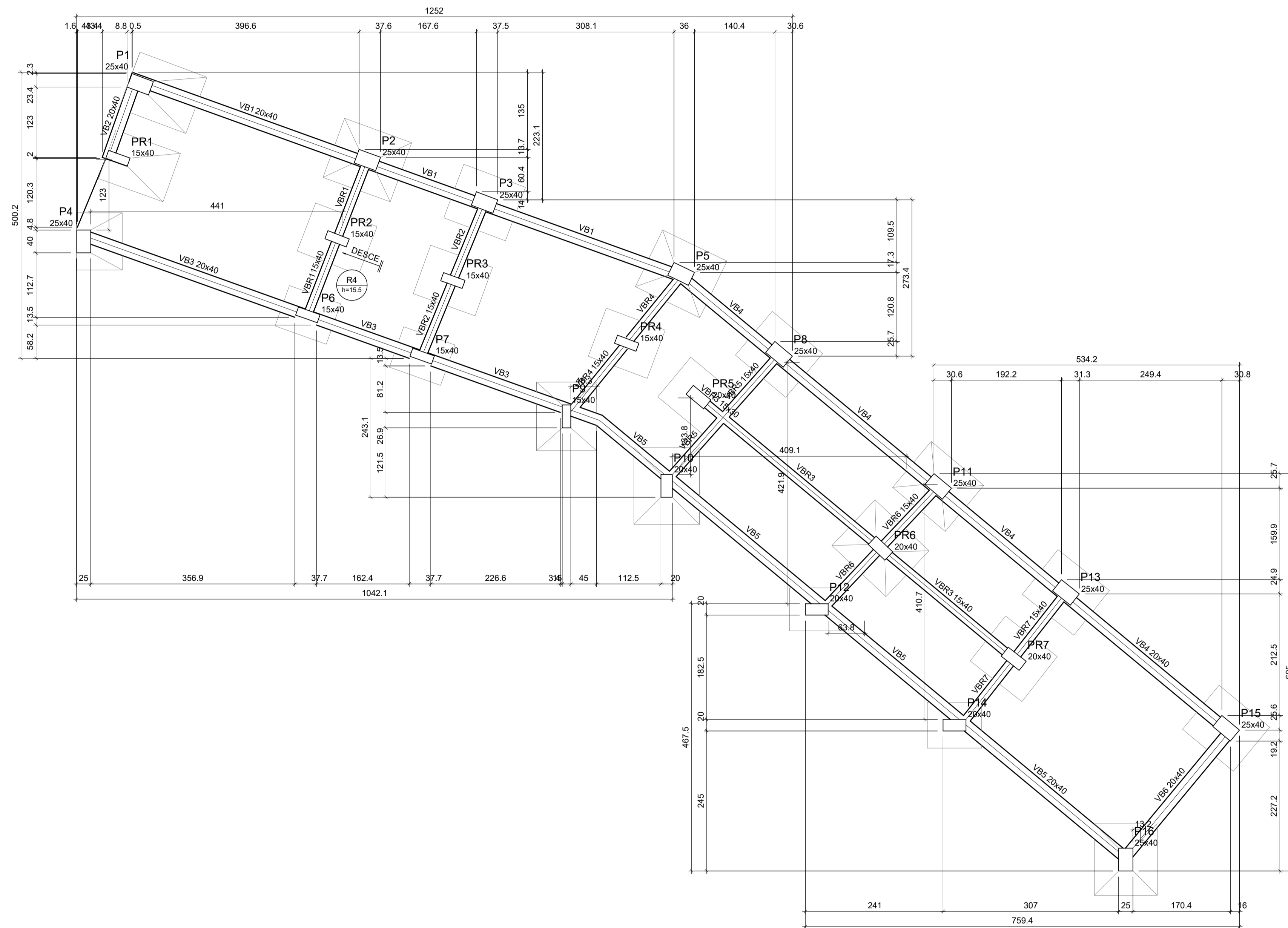
Forma do pavimento Fundação (Nível 0)
