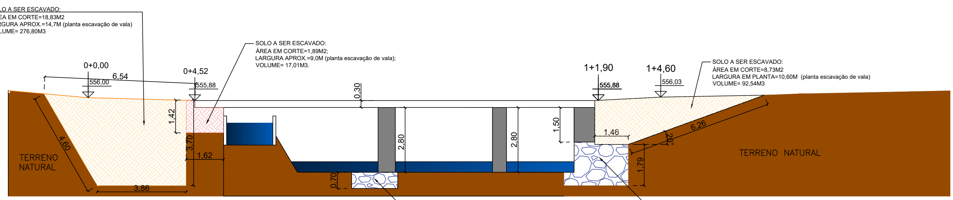
Corte Longitudinal - Volume escavação ESCALA: 1/100
