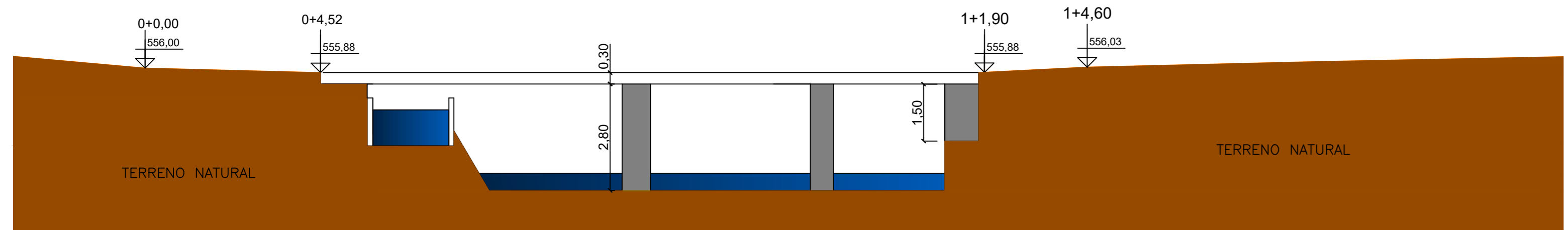
Corte Longitudinal da Ponte existente ESCALA: 1/100
