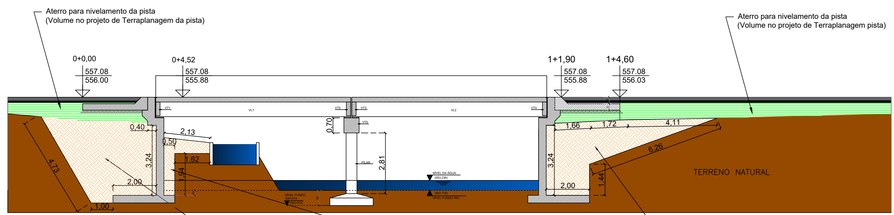
Corte Longitudinal - Reaterro ESCALA: 1/100
