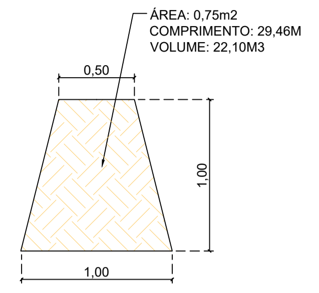
Corte transversal: Ensecadeira ESCALA: 1/25
