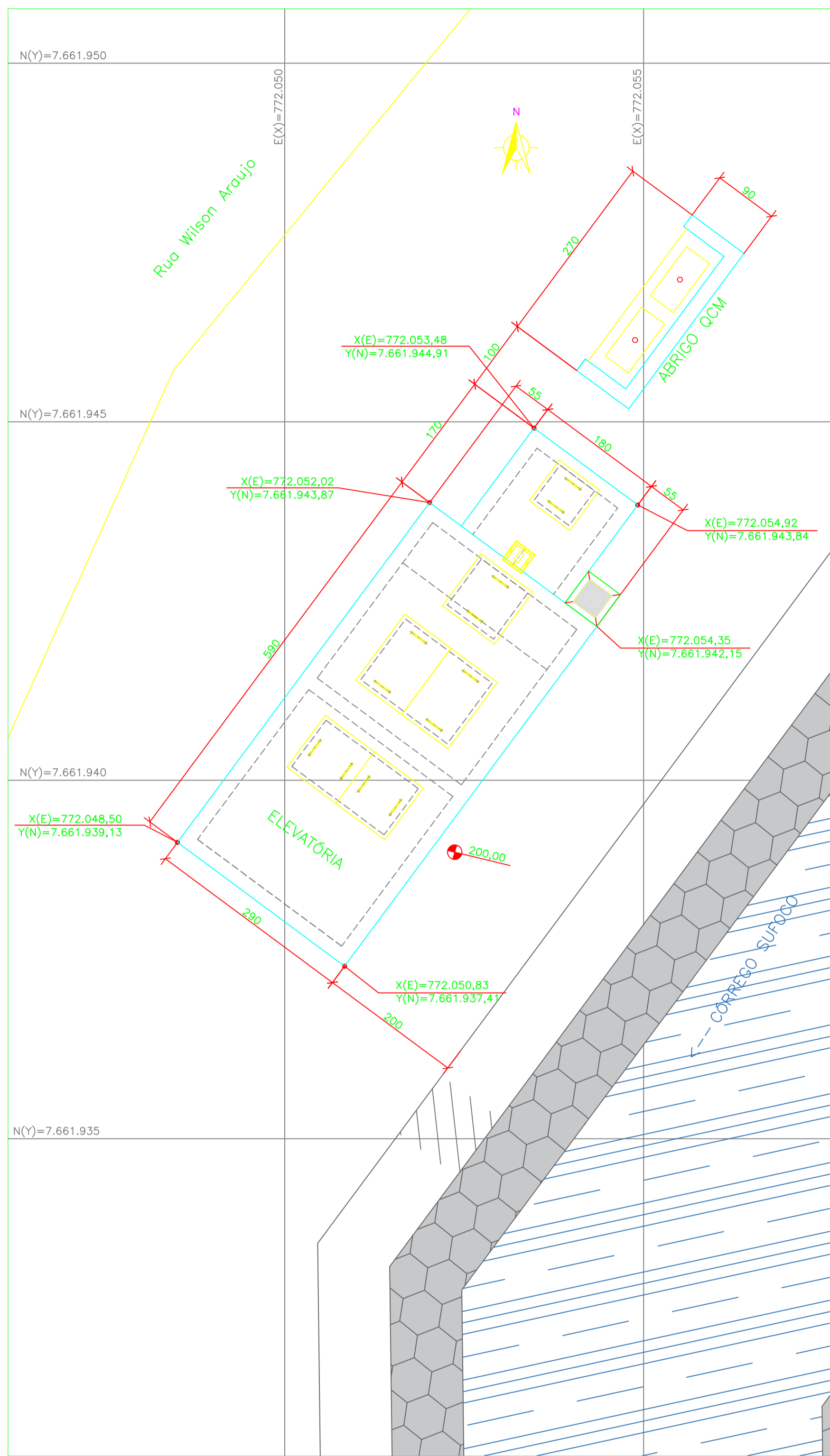
PLANTA LOCALIZAÇÃO ESC.: 1:50
