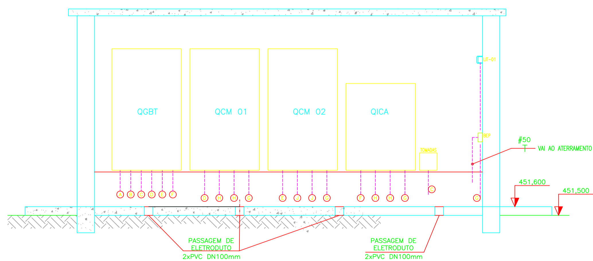
ABRIGO DO QCM - VISTA FRONTAL ESC. 1:25
