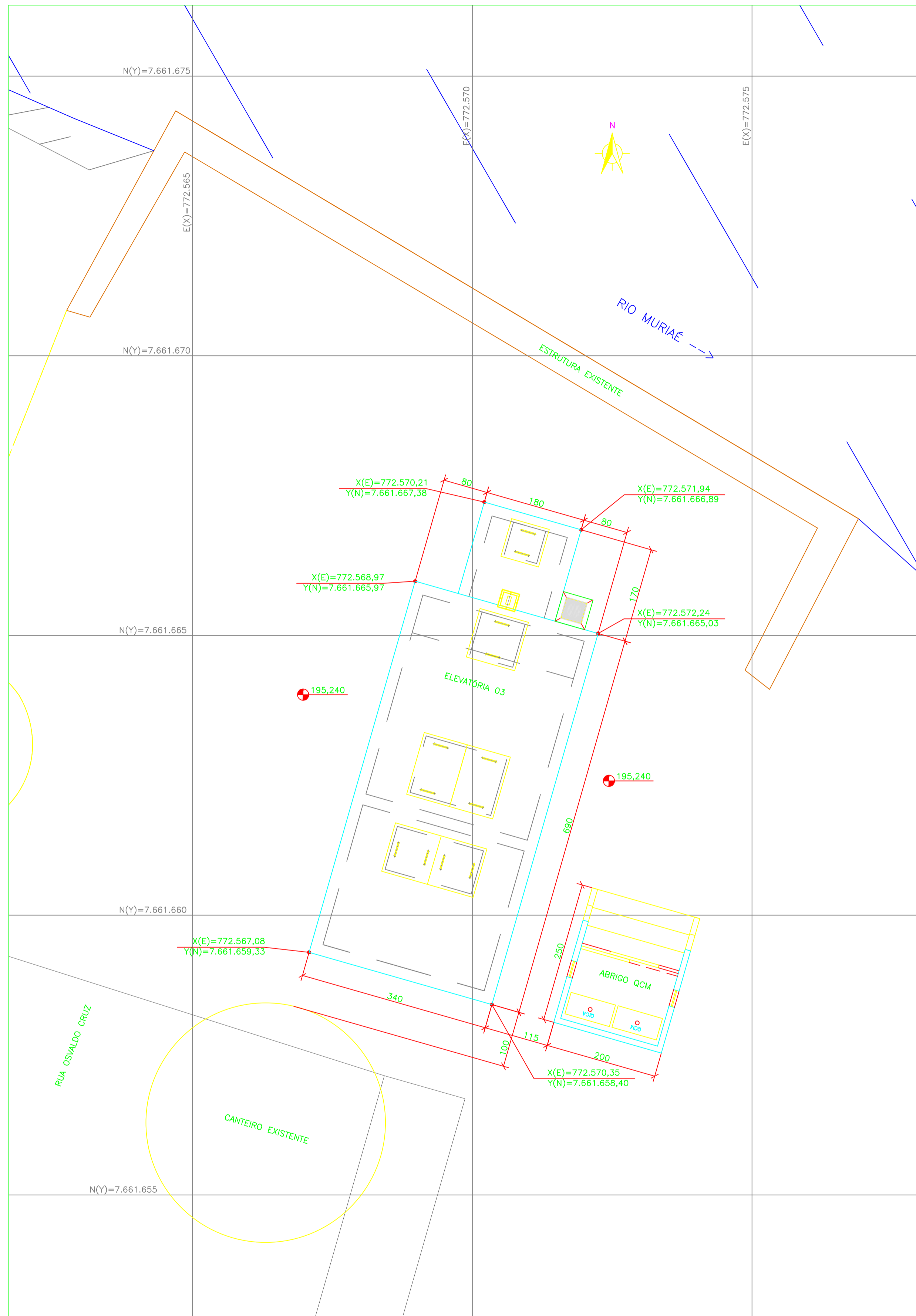
LOCAÇÃO ELEVATÓRIA 03 ESC.: 1:50
