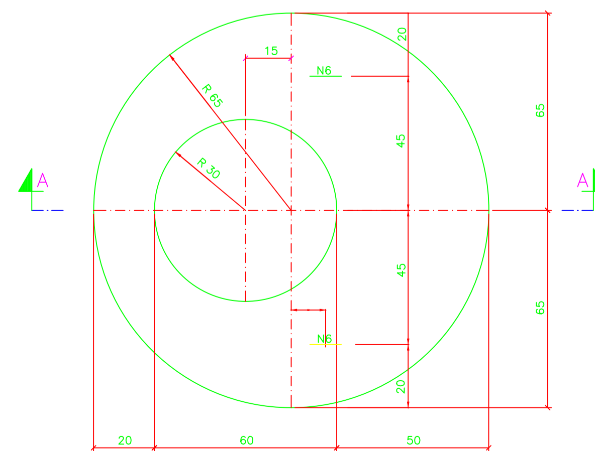
LAJE DE REDUÇÃO ESC.: SEM ESC.
