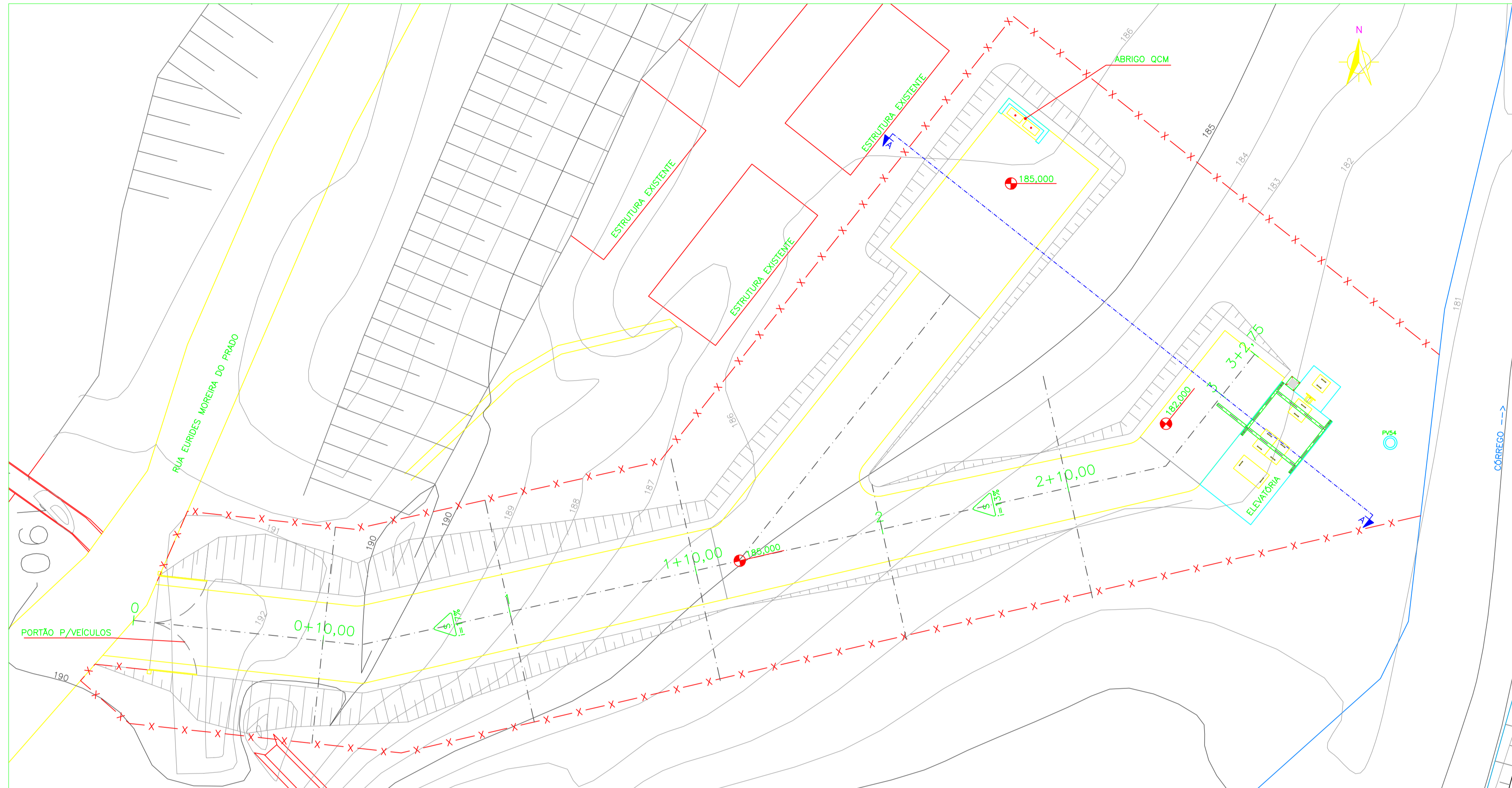
PLANTA DE TERRAPLENAGEM ESC.: 1:150
