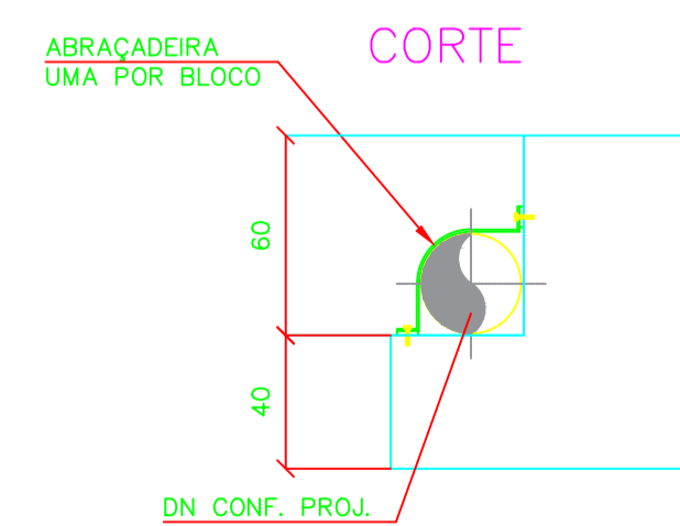
BLOCO DE ANCORAGEM PARA CURVA 90°
