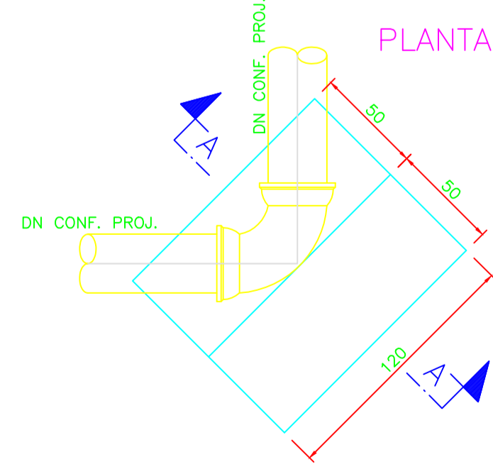
BLOCO DE ANCORAGEM PARA CURVA 90°
