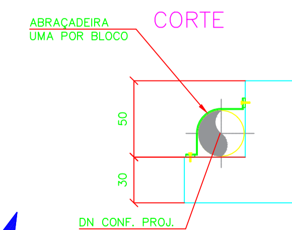
ABRACADEIRA UMA POR BLOCO
