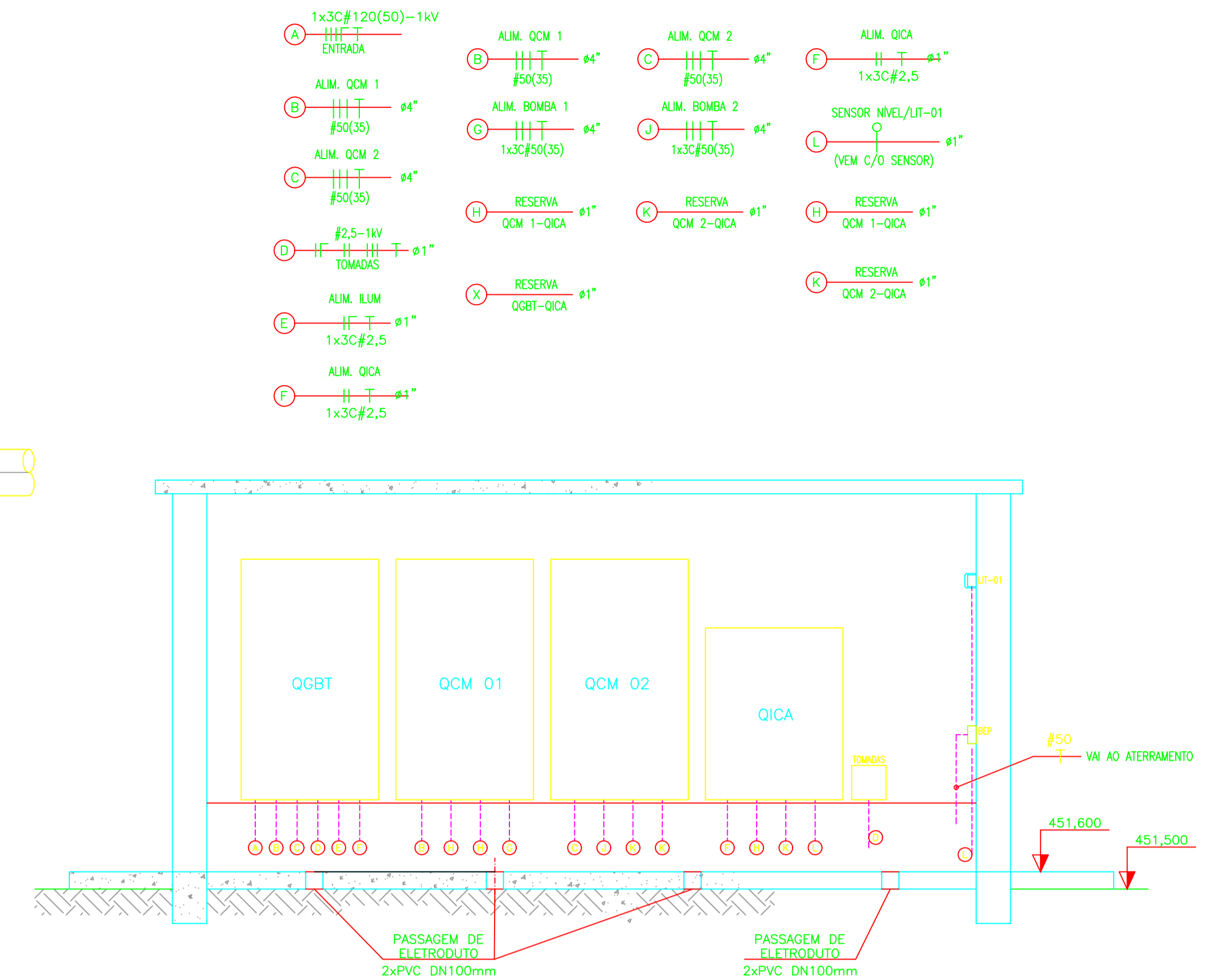
ABRIGO DO QCM - VISTA FRONTAL ESC. 1:25
