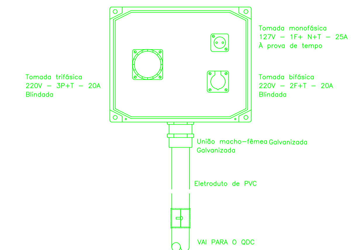
DETALHE TÍPICO DE TOMADA PARA MANUTENÇÃO
