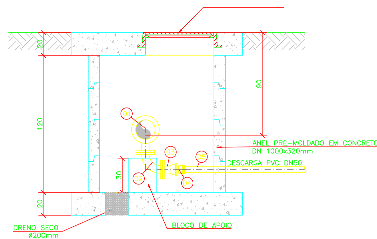
CAIXA DE DESCARGA CORTE A-A
