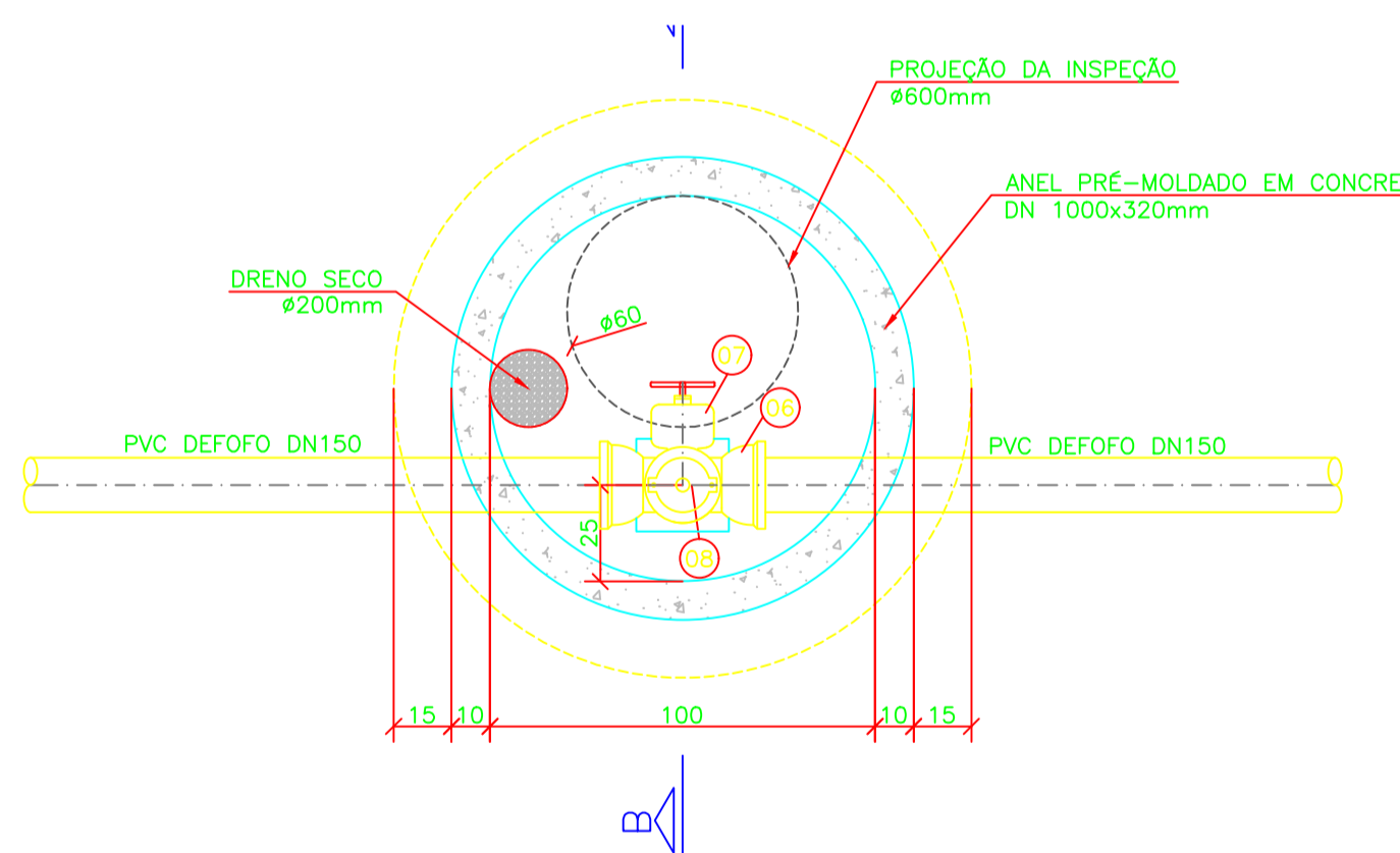
CAIXA DE VENTOSA PLANTA
