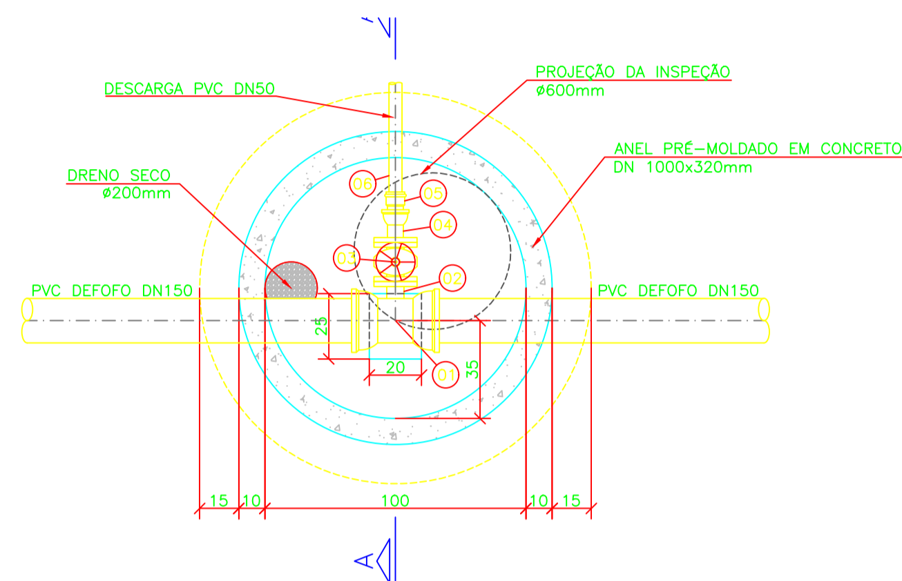
CAIXA DE DESCARGA PLANTA
