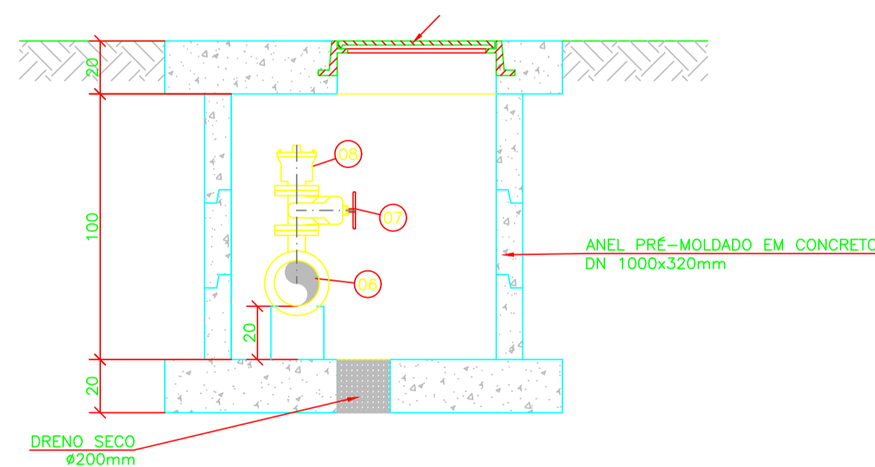
CAIXA DE VENTOSA CORTE B-B
