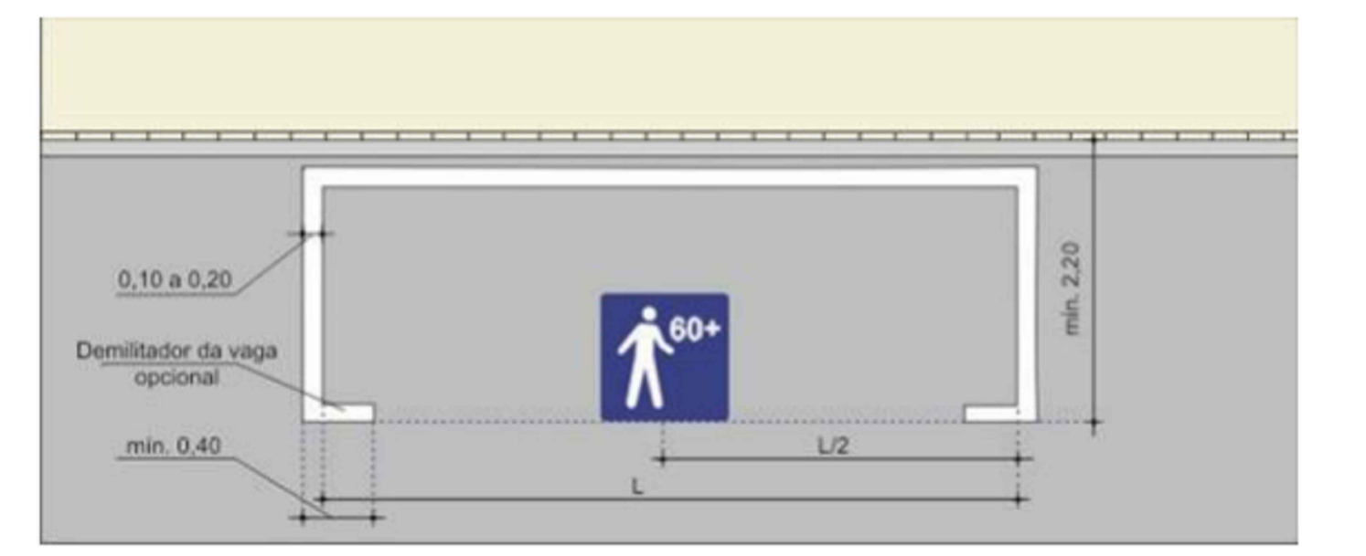
DETALHE TÍPICO: VAGA IDOSO SEM ESCALA
