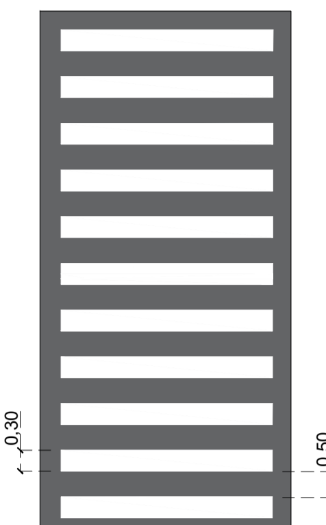
DETALHE TÍPICO: FAIXA DE PEDESTRES ESCALA 1/100
