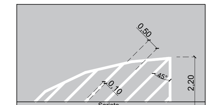
DETALHE TÍPICO: ÁREA DE PAVIMENTO NÃO UTILIZÁVEL ESCALA 1/100
