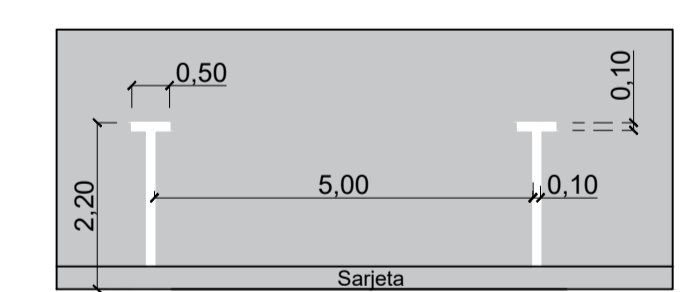
DETALHE TÍPICO: VAGA DE ESTACIONAMENTO ESCALA 1/100
