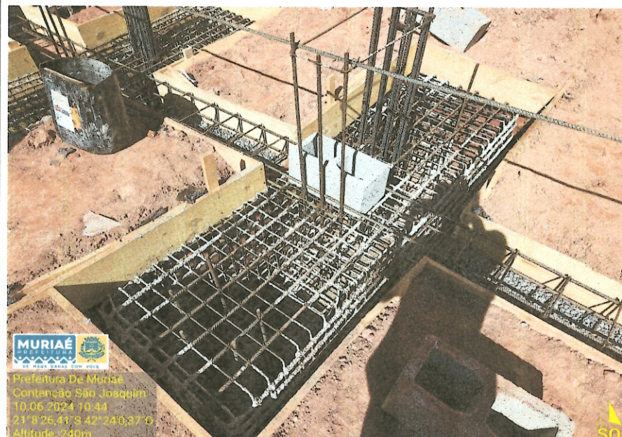
Figura 18 - Fabricação, montagem e desmontagem de formas para blocos de coroamento e viga baldrame
