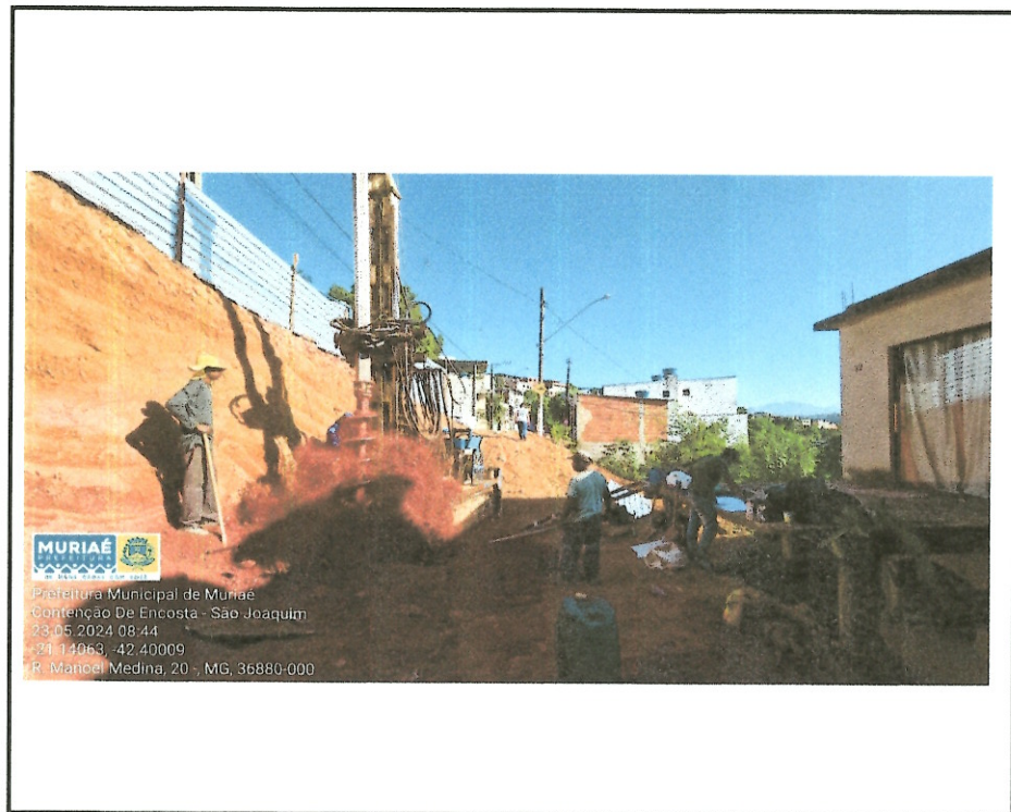
Figura 12 - Estaca escavada mecanicamente 40 cm de diâmetro e concretagem
