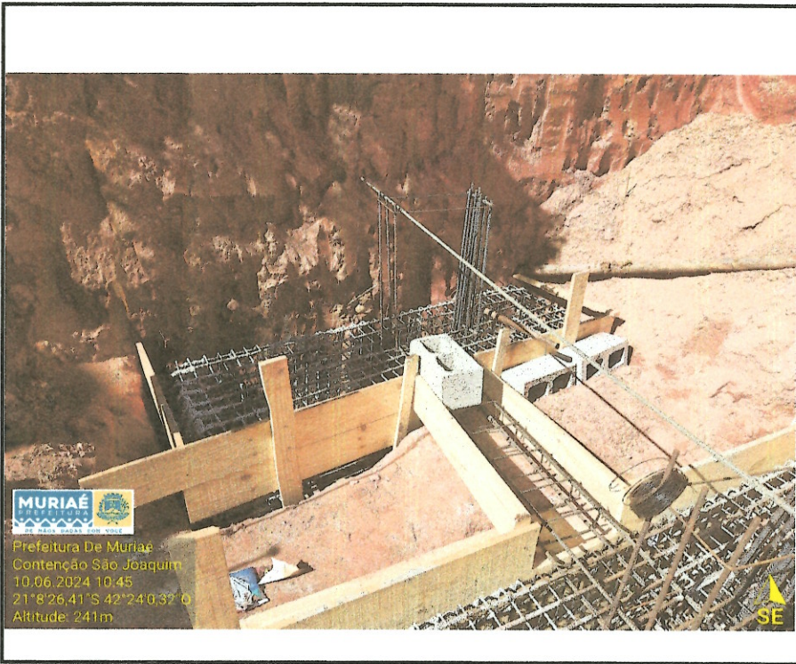
Figura 19 - Fabricação, montagem e desmontagem de formas para blocos de coroamento e viga baldrame
