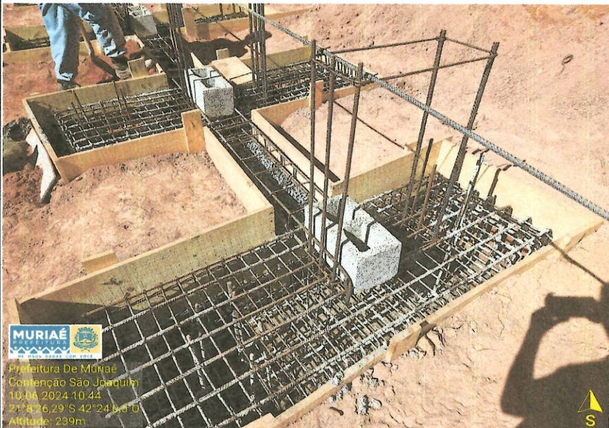
Figura 17 - Fabricação, montagem e desmontagem de formas para blocos de coroamento e viga baldrame
