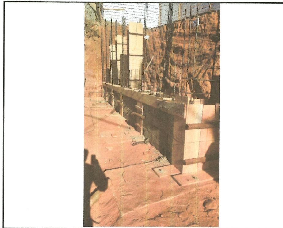
Figura 26 - Corte, dobra e montagem de aço CA-50 e fabricação de formas para vigas
