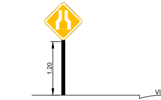
DETALHE- A21-A SINALIZAÇÃO VERTICAL ESCALA: 1:50
