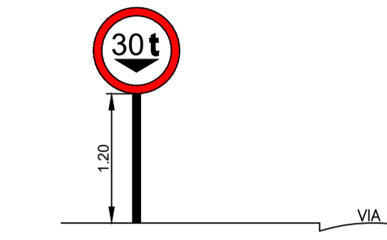
DETALHE- R14 SINALIZAÇÃO VERTICAL ESCALA: 1:50
