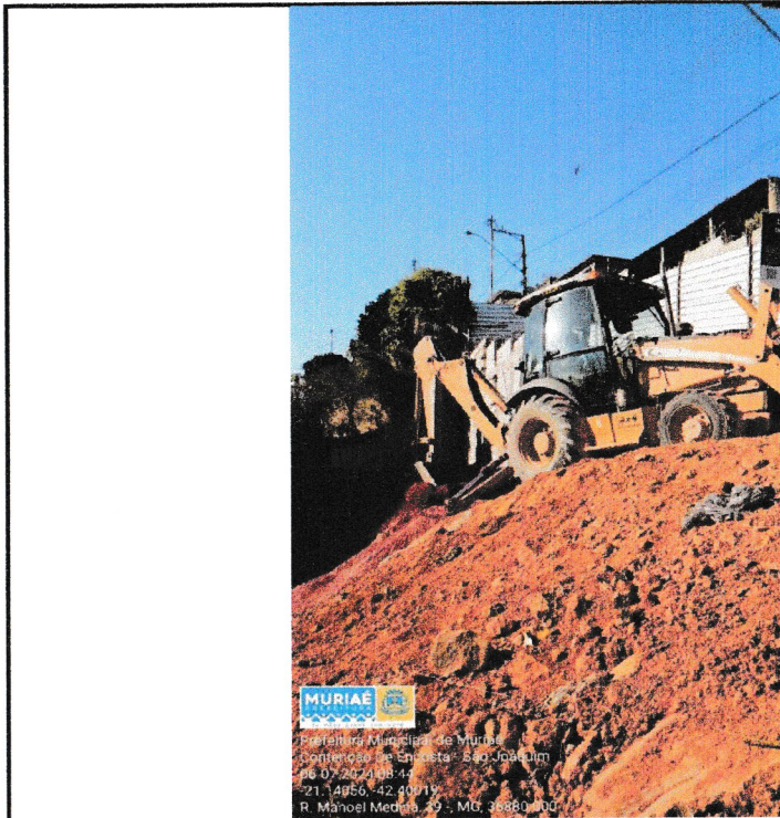
Figura 05 - Escavação vertical, carga e transporte de solo de 1ª categoria
