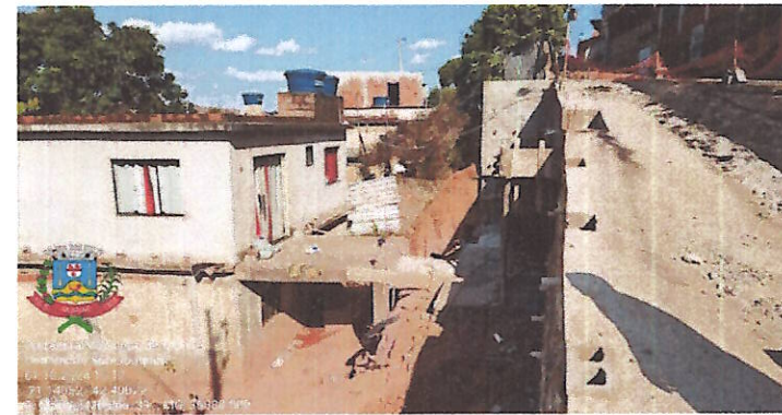
Figura 14 - Execução de estrutura de escada (baldrames e pilares)
