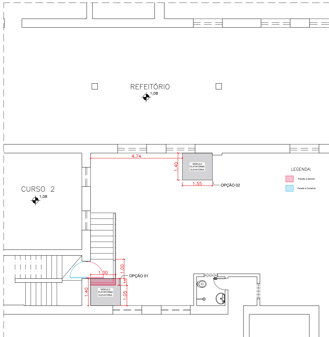
PLANTA BAIXA DEMOLIR/CONSTRUIR - PAVIMENTO TÉRREO - PLATAFORMA ELEVATÓRIA - DOM DELFIM ESC 1:100
