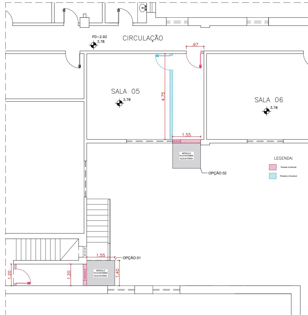
PLANTA BAIXA DEMOLIR/CONSTRUIR - SEGUNDO PAVIMENTO - PLATAFORMA ELEVATÓRIA - DOM DELFIM ESC 1:100
