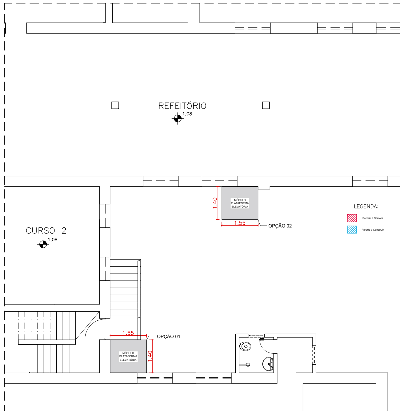
PLANTA BAIXA PROJETO - PAVIMENTO TÉRREO - PLATAFORMA ELEVATÓRIA - DOM DELFIM ESC 1:100
