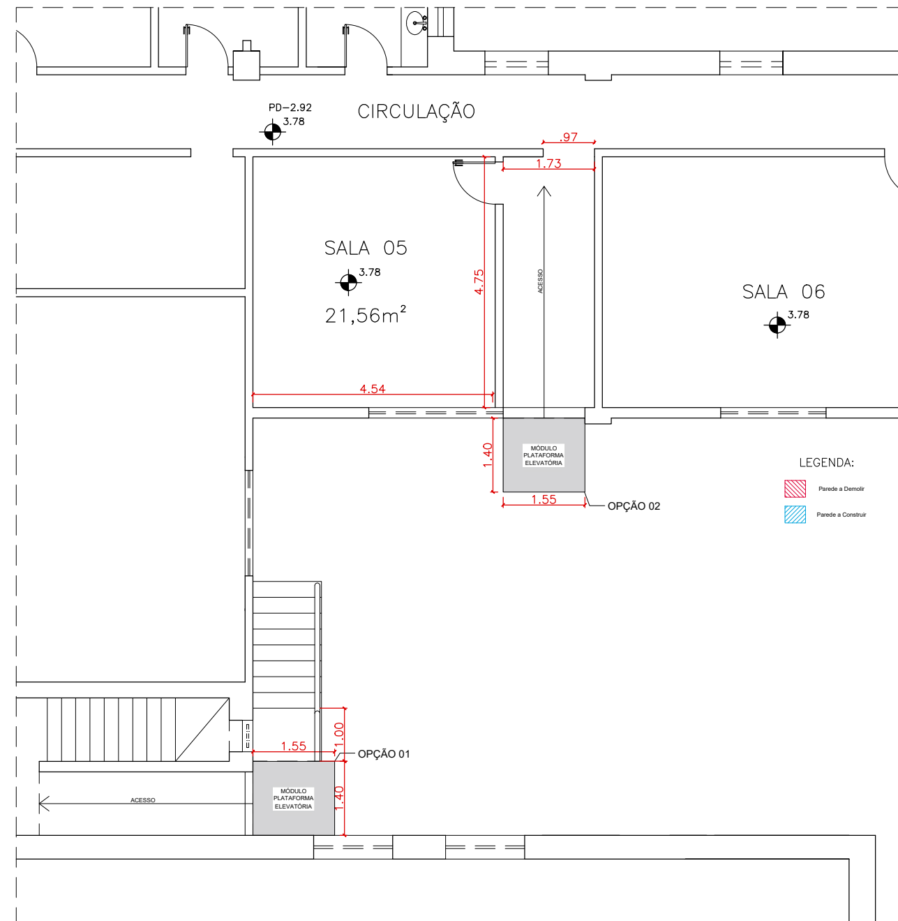
PLANTA BAIXA PROJETO - SEGUNDO PAVIMENTO - PLATAFORMA ELEVATÓRIA - DOM DELFIM ESC 1:100
