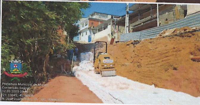
Figuras 5 e 6 - Escavação de drenagem de pé com brita, separação do drenagem do entulho, compactação dos sacos de areia e cimento
