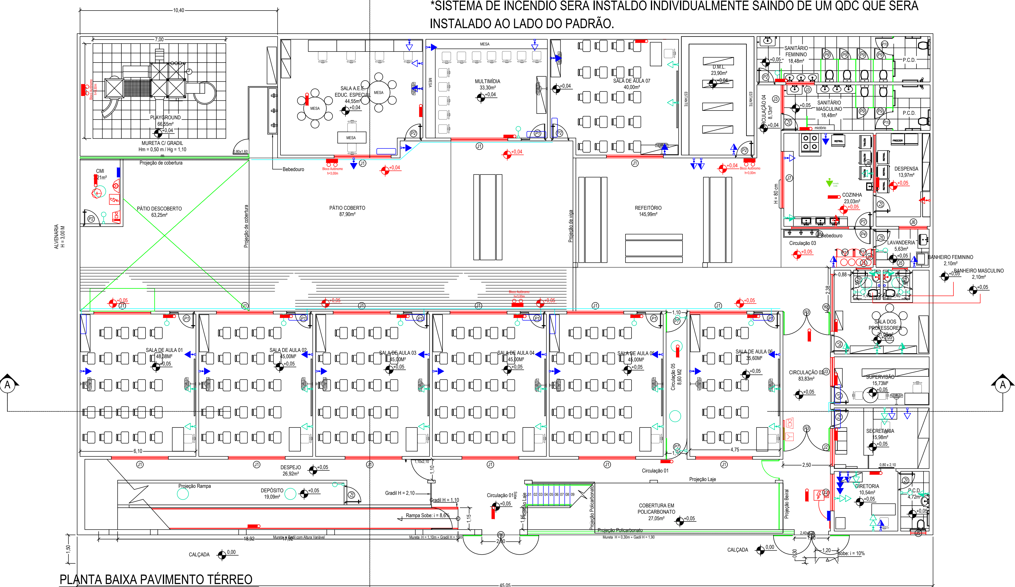
PLANTA BAIXA PAVIMENTO TÉRREO ÁREA: 1.069,48m² ESCALA: 1/100
