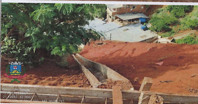
Figuras 13 e 14: Escada hidráulica em concreto armado
