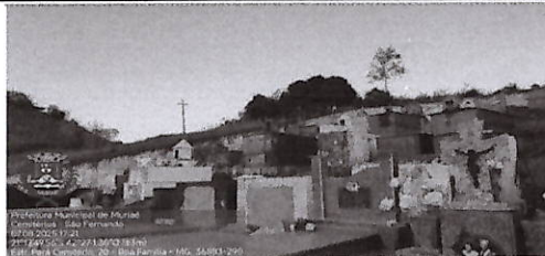
IMAGEM 3: MURO LATERAL INFERIOR DANIFICADO LOCAL: CEMITÉRIO DE SÃO FERNANDO
