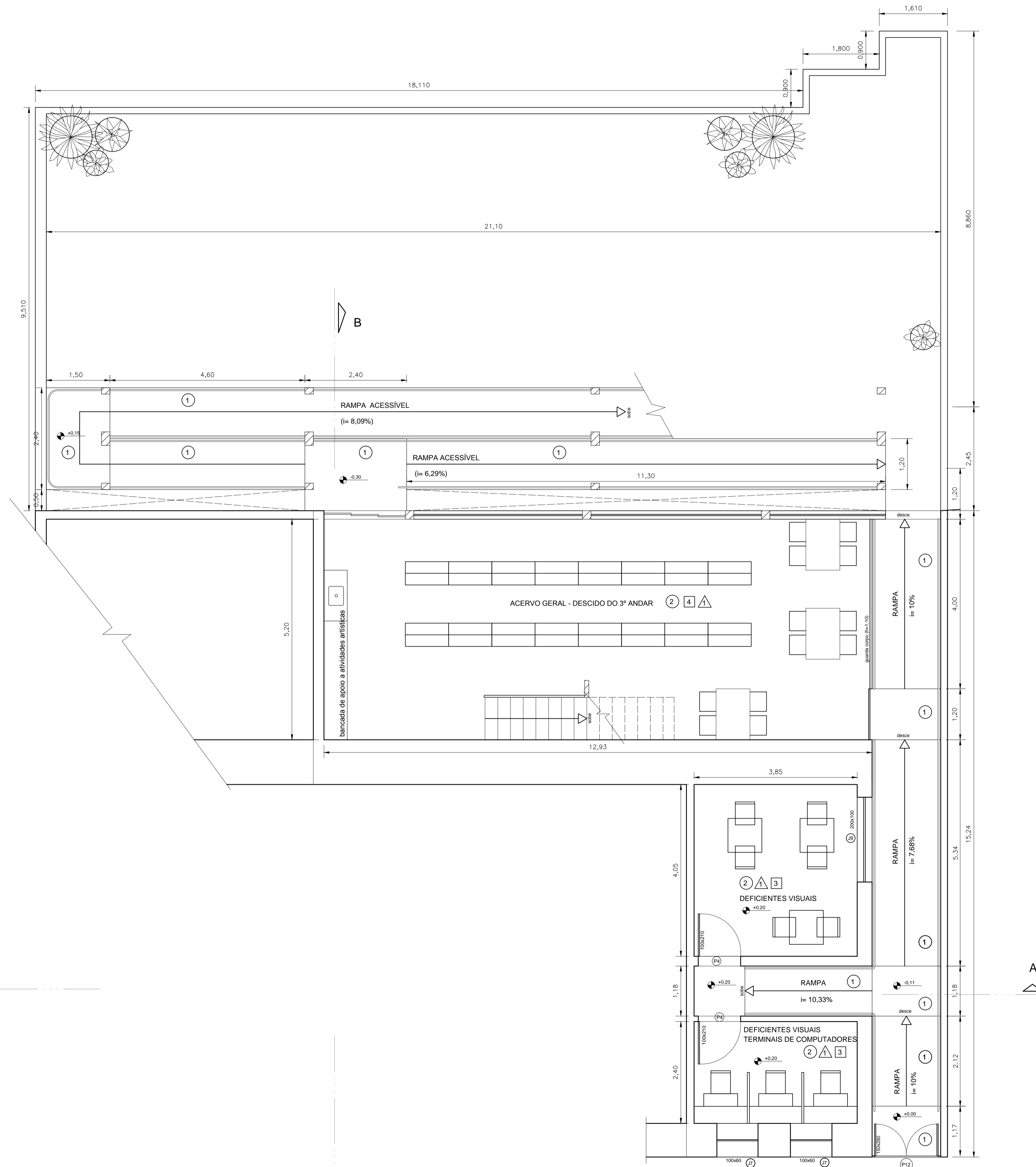
PLANTA BAIXA - SUBSOLO ESCALA 1 : 100
