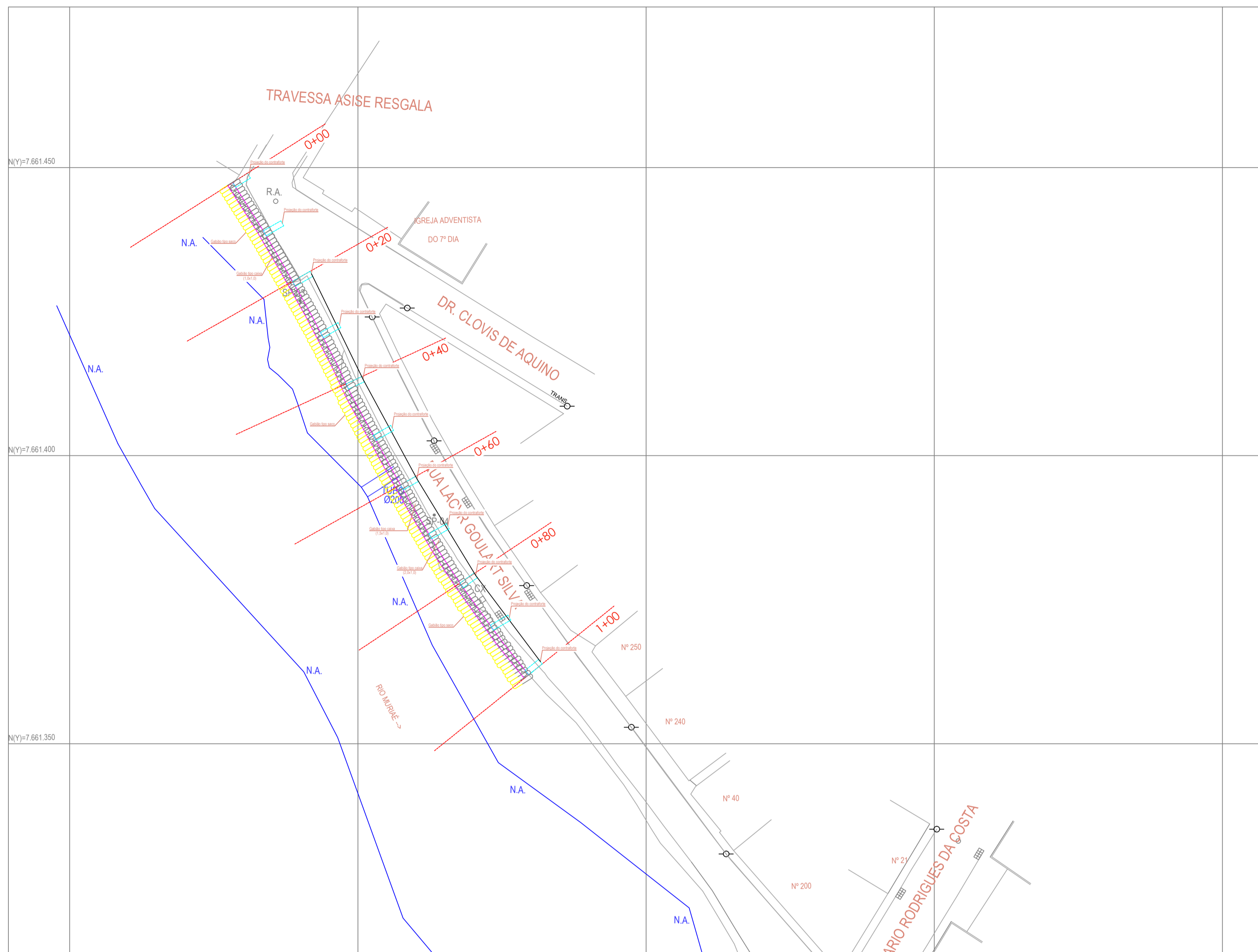
PLANTA BAIXA - LOCAÇÃO DA CONTENÇÃO E ESTAQUEAMENTO ESC: 1/500
