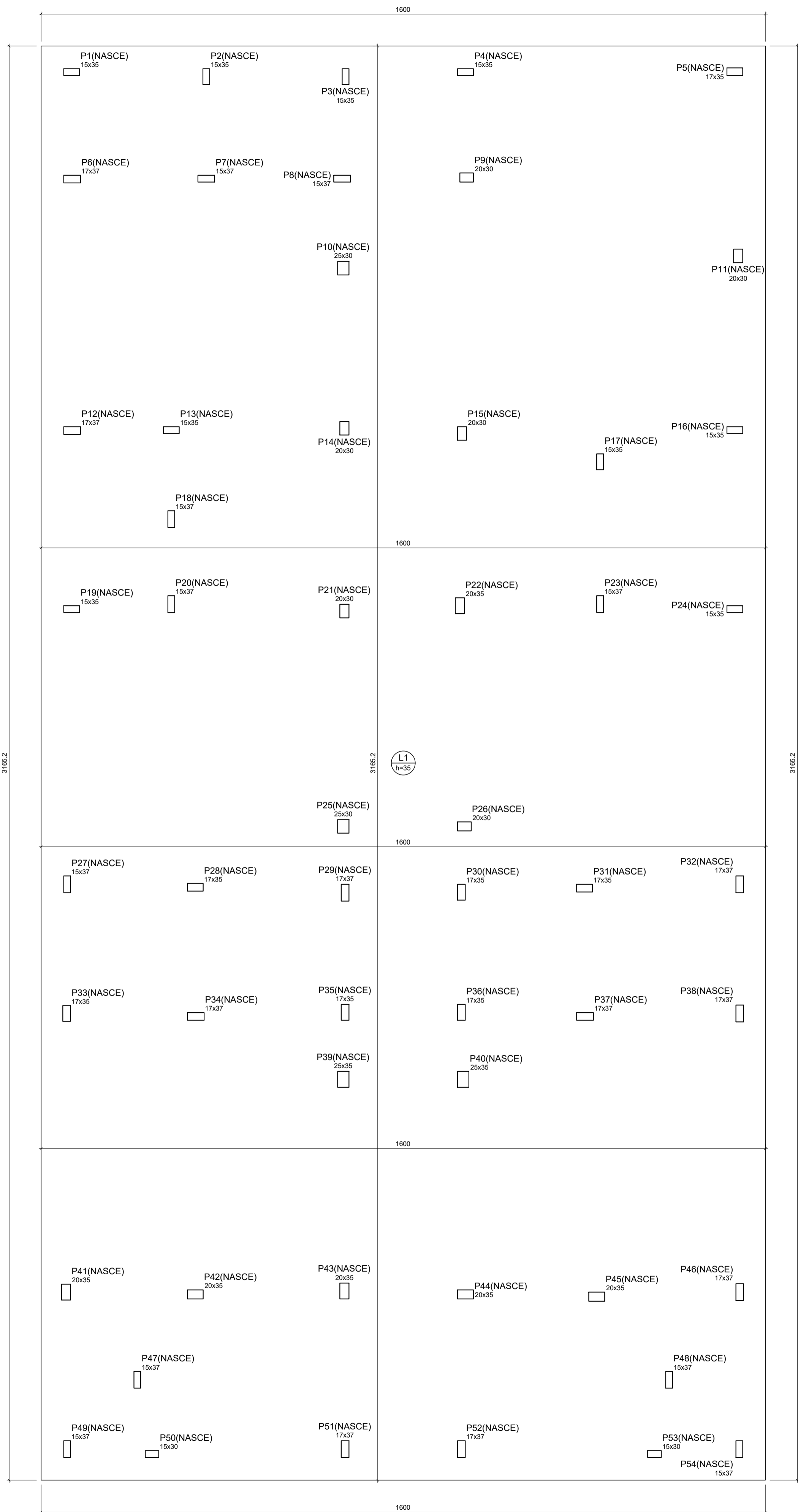
Forma do pavimento Fundação (Nível 0)
