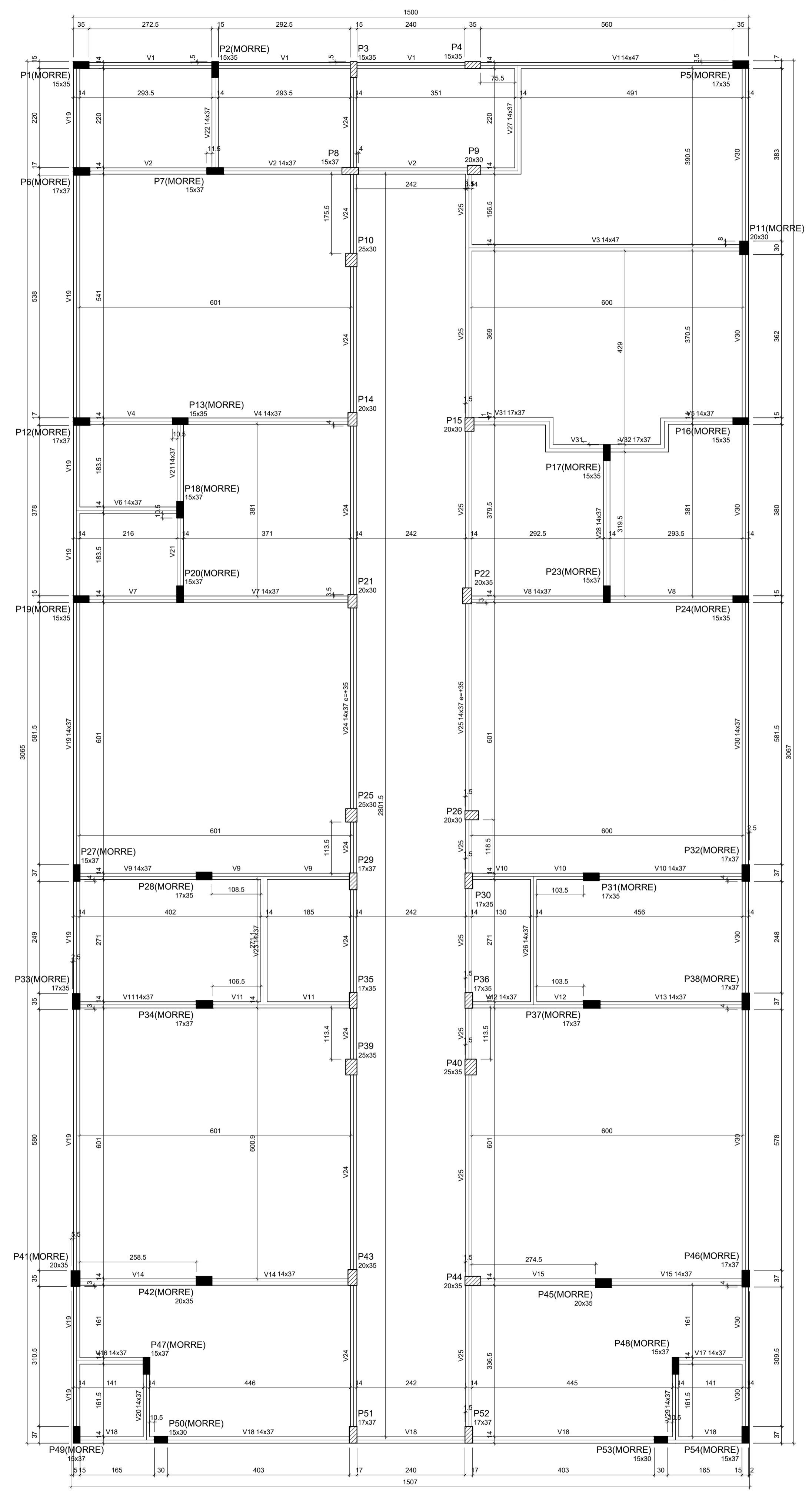
Forma do pavimento Terreo (Nível 337) escala 1:50
