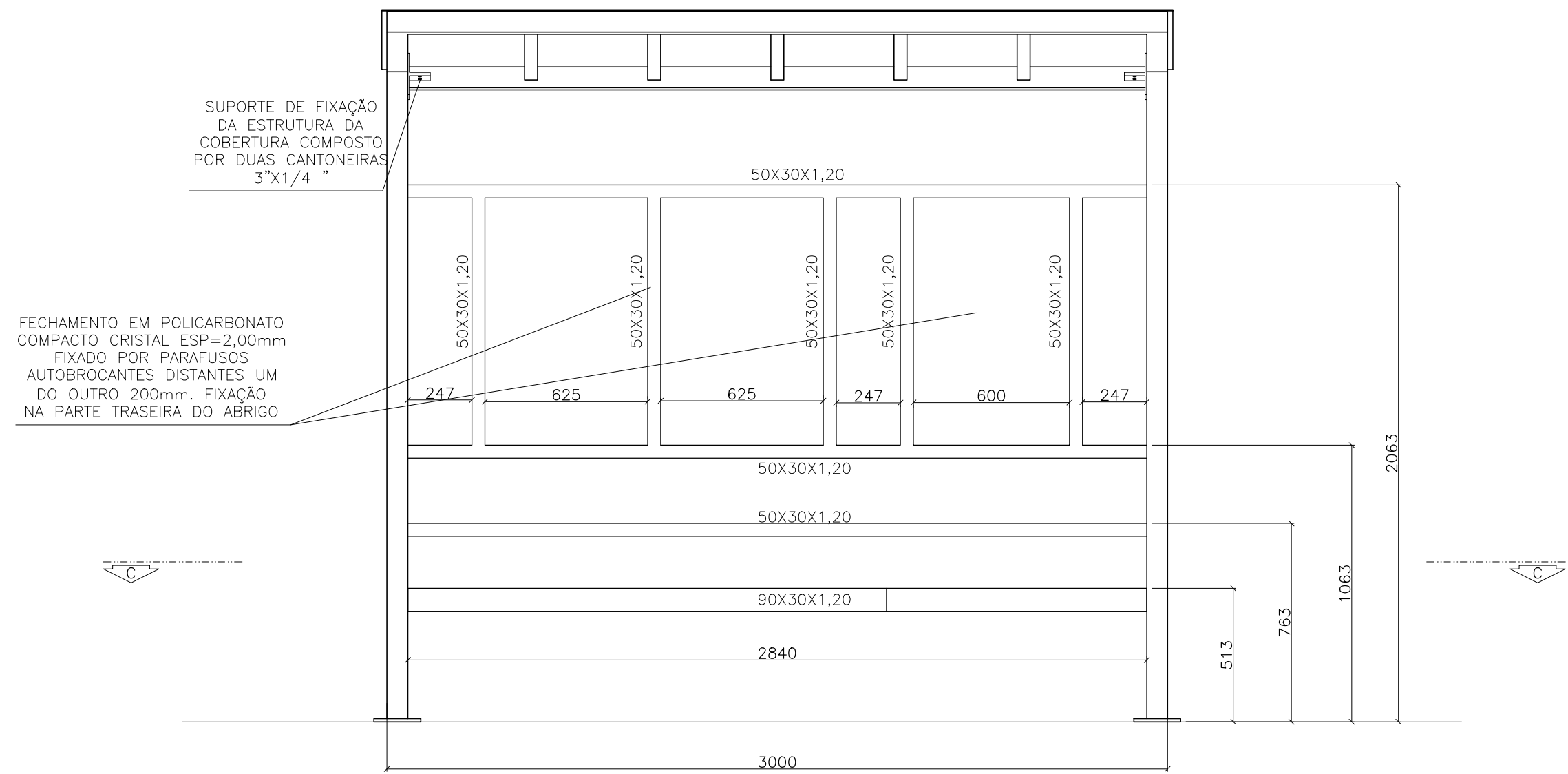
VISTA FRONTAL DO ABRIGO COM MODIFICAÇÃO PARA PORTADORES DE NECESSIDADES ESPECIAIS esc 1:20
