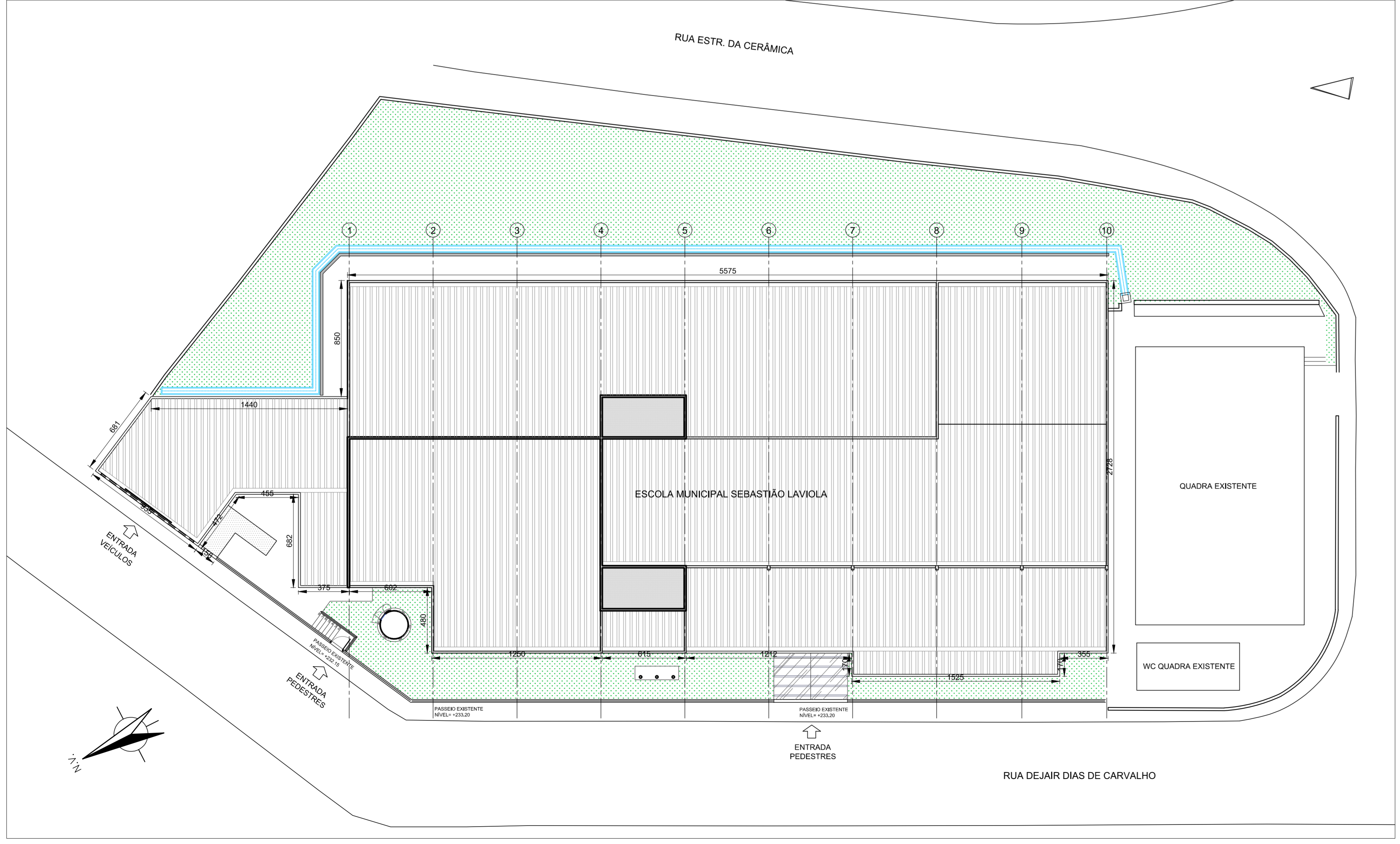
PLANTA DE LOCALIZAÇÃO ESCALA - 1/200
